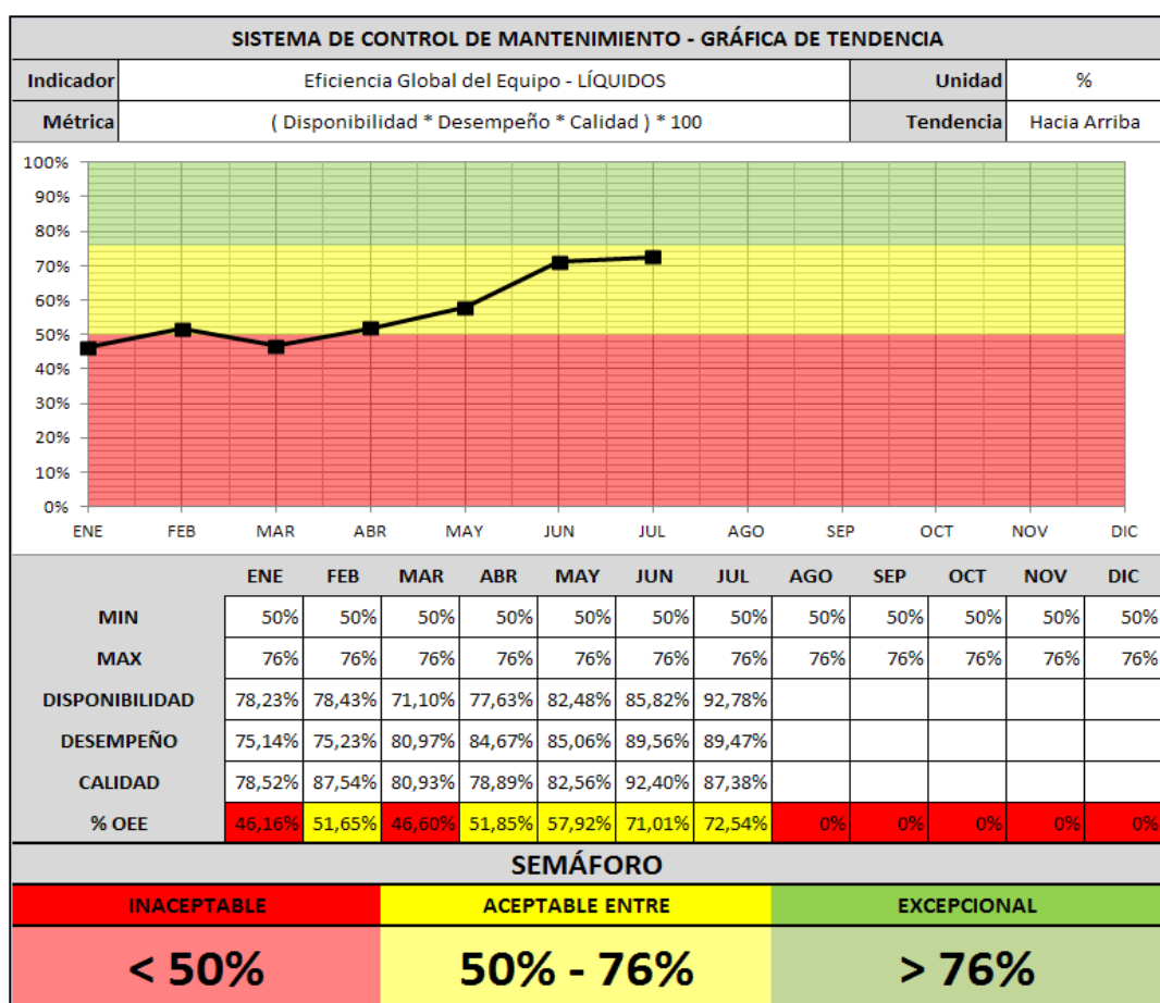
FIGURA 4.16. GRÁFICA DE TENDENCIA N°3 - INDICADOR OEE LÍQUIDOS
