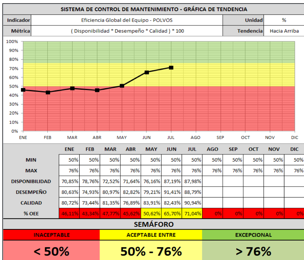
FIGURA 4.15. GRÁFICA DE TENDENCIA N°2 - INDICADOR OEE POLVOS
