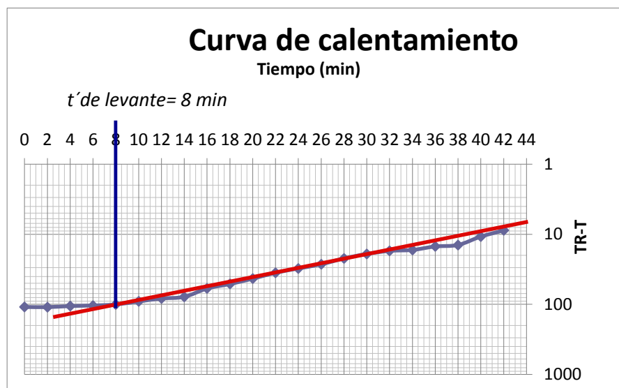
FIGURA 3. 5. GRÁFICO DE DATOS DE CALENTAMIENTO CÁLCULO DE “t pi ”
