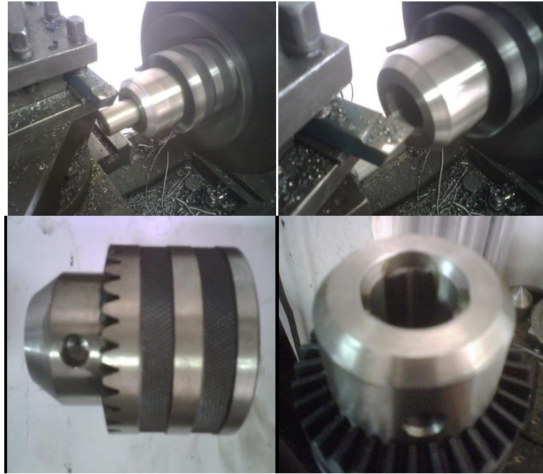
FIG. 2.8 PROCESO DE MECANIZADO DE LOS MANDRILES DE SUJECCIÓN
