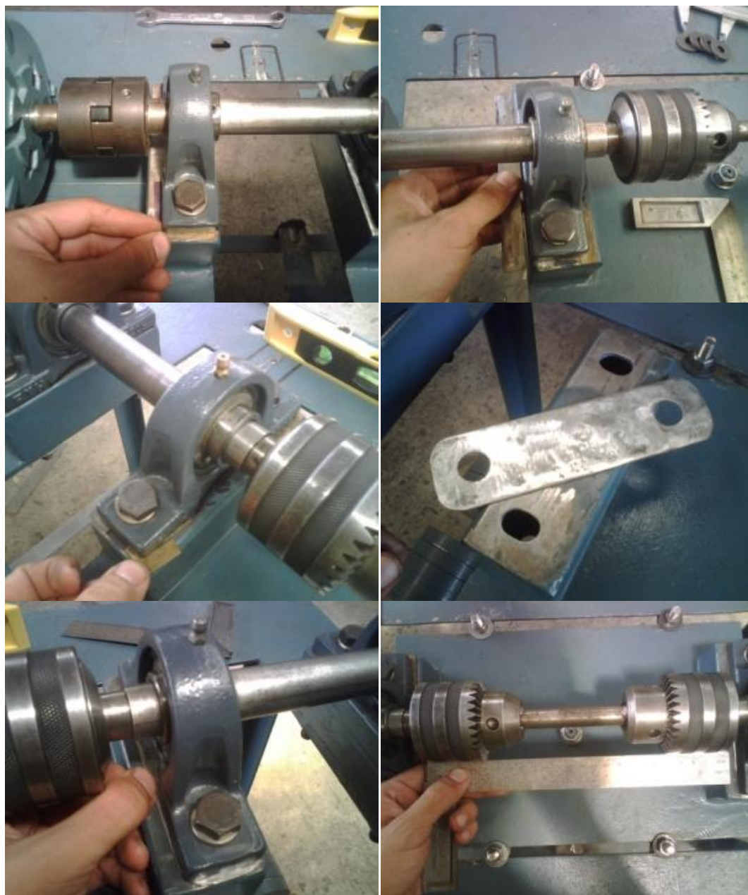
FIG. 2.29 PROCESO DE CALIBRACIÓN Y PUESTA A PUNTO DEL DISPOSITIVO (CONTINUACIÓN)
