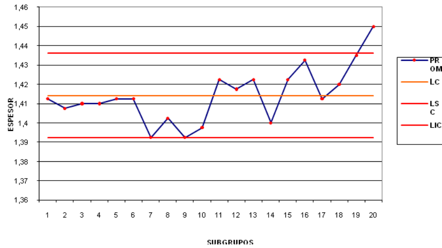
FIGURA 4.22. GRÁFICO DE CONTROL DE ESPESOR ZONA B
