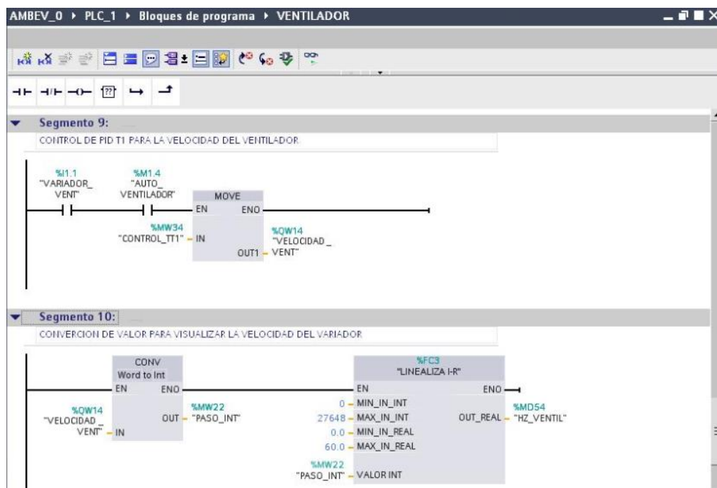
Figura 16. Ejemplo de programa del ventilador
