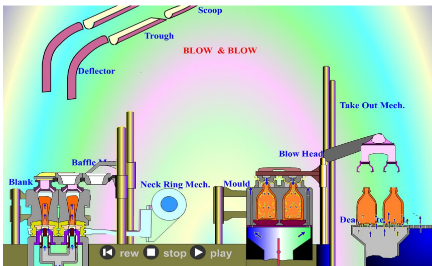
Fig. 1.2 Proceso de formación Soplo & Soplo.
