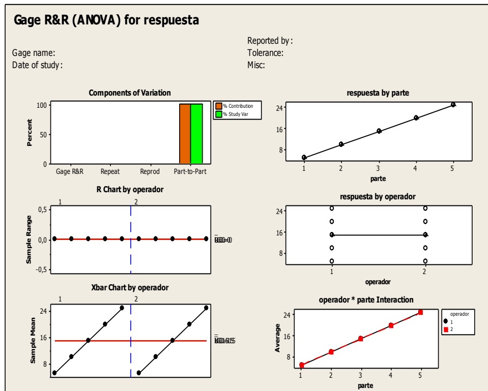
Fig. 3.5 Prueba R&R del sistema de medición.
