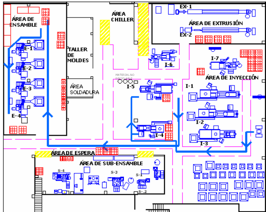
FIGURA 2.14 RECORRIDO DE LA TAPA
