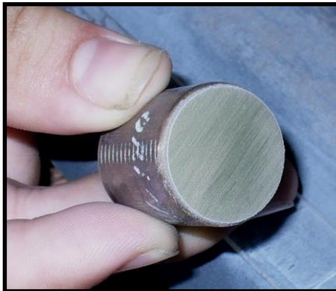
FIGURA 2.2 PROBETA DE BRONCE SAE 64 PARA HOMOLOGAR
