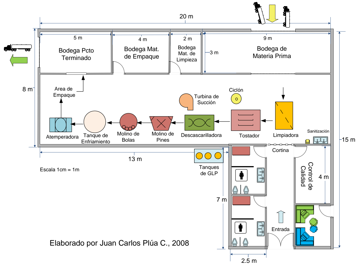
FIGURA 3.5 LAYOUT DE LA PLANTA
