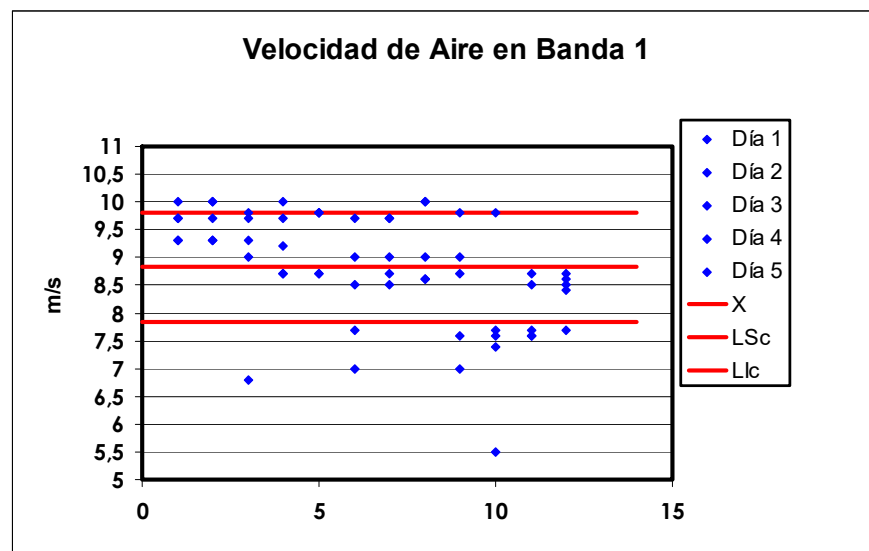
Figura 4.1 Gráfica de Control de VELOCIDAD DE AIRE en banda 1 del túnel de congelación
