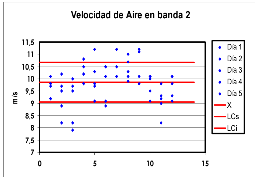
Figura 4.2 Gráfica de Control de VELOCIDAD DE AIRE en banda 2 del túnel de congelación
