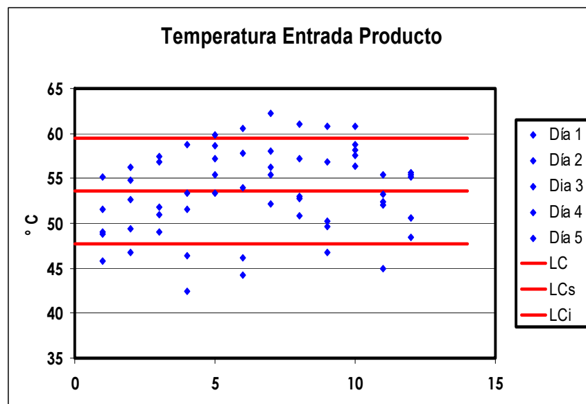
Figura 4.4 Gráfica de Control de TEMPERATURA DE ENTRADA DEL PRODUCTO al túnel de congelación
