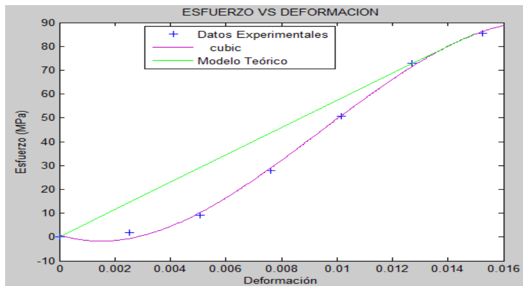
FIGURA 30 MODELACION (DIA 28 - MUESTRA 1 - 15%)
