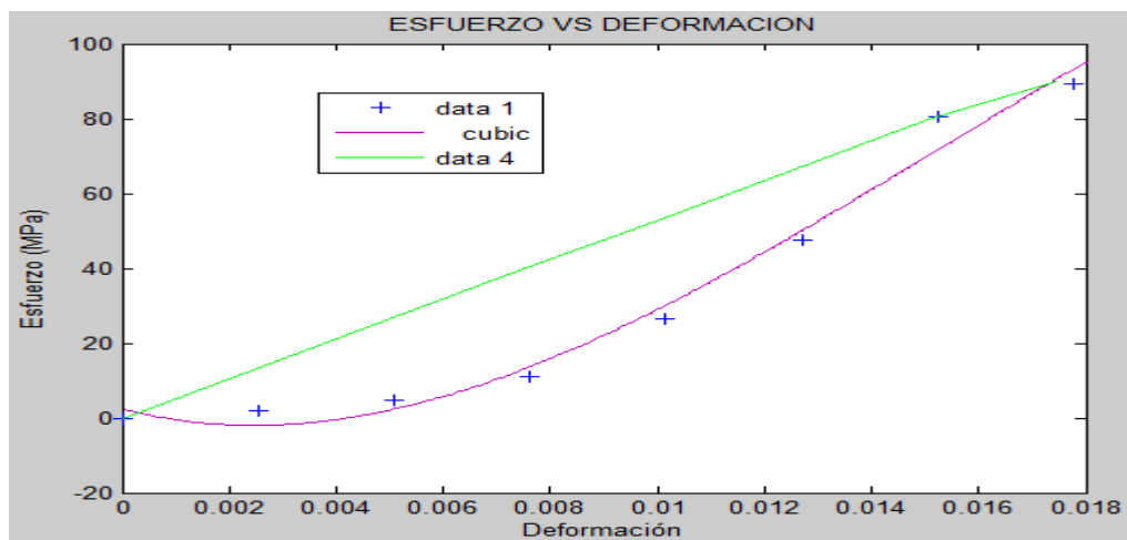
FIGURA 18 MODELACION (DIA 25 - MUESTRA 1 - 17.5%)
