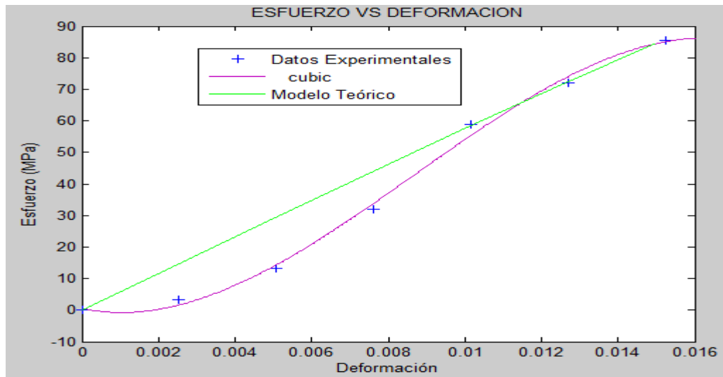
FIGURA 29 MODELACION (DIA 21 - MUESTRA 3 - 15%)
