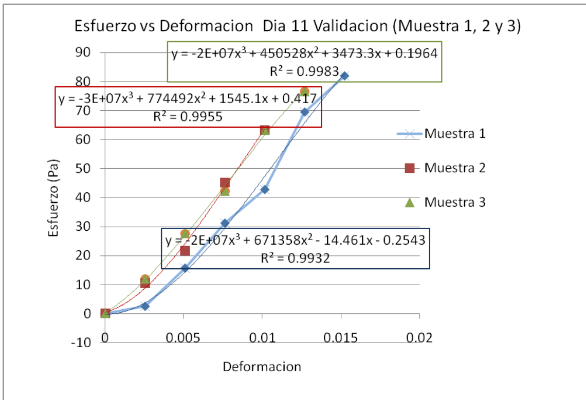
FIGURA 2 ESFUERZO VS DEFORMACION DIA 11
