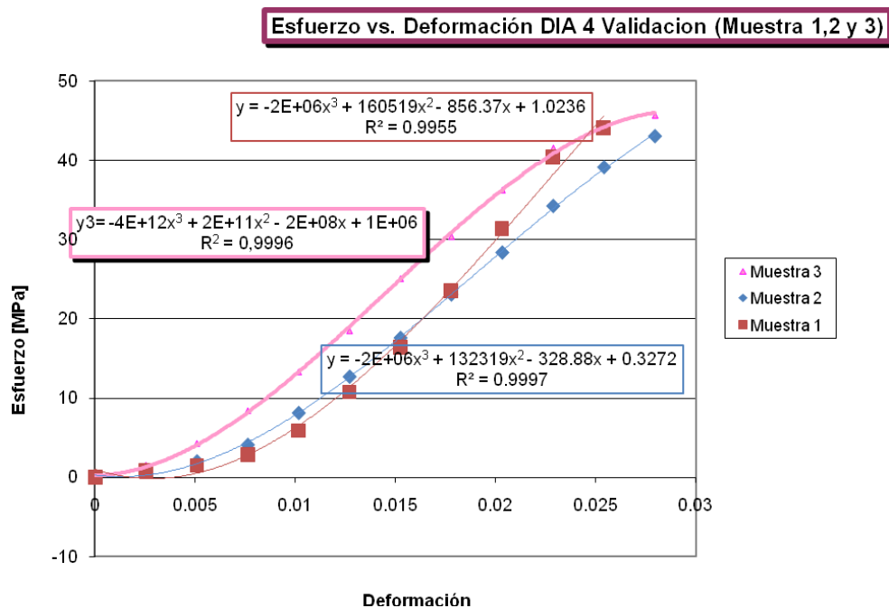
FIGURA 1 ESFUERZO VS DEFORMACION DIA 4
