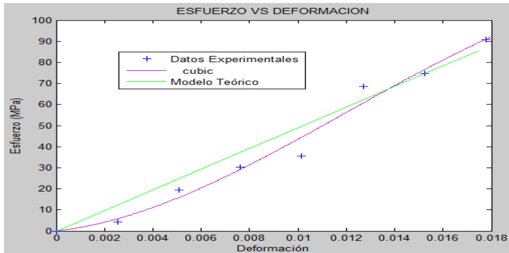
FIGURA 25 MODELACION (DIA 14 - MUESTRA 2 - 15%)
