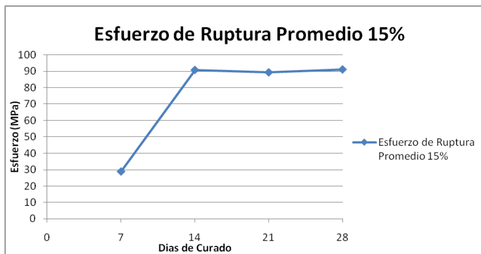
FIGURA 4.1 GRAFICA ESFUERZO DE RUPTURA EXPERIMENTACION
