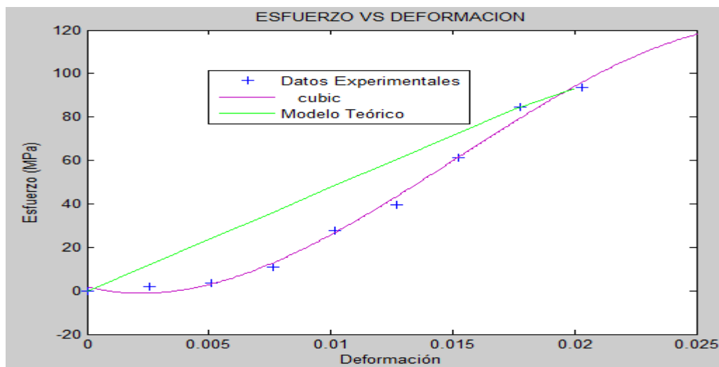
FIGURA 28 MODELACION (DIA 21 - MUESTRA 2 - 15%)
