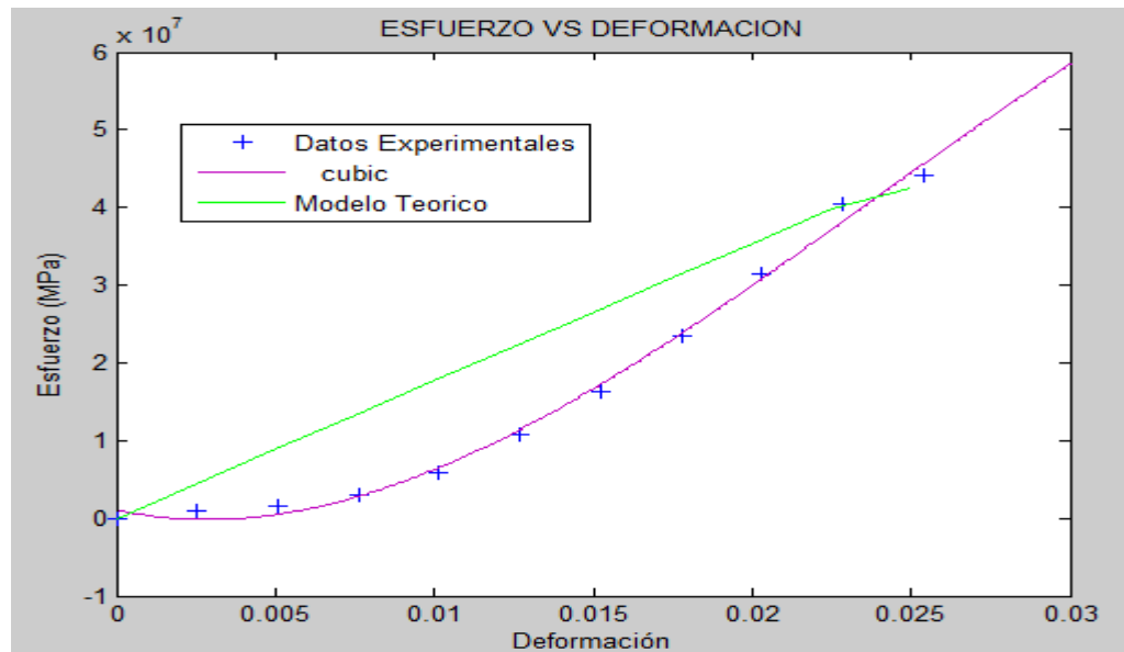
FIGURA 9 MODELACION (DIA 4 - MUESTRA 1 - 17.5%)
