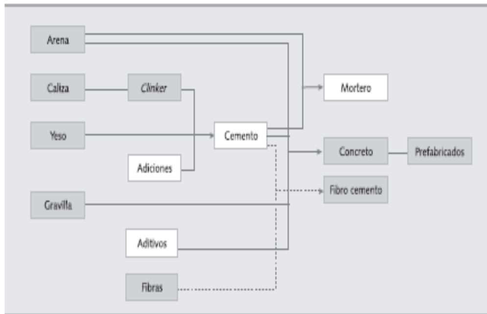
Figura 2.1.- ESTRUCTURA SIMPLIFICADA DEL CEMENTO [2]
