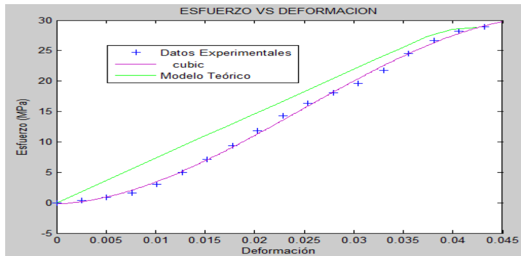
FIGURA 22 MODELACION (DIA 7 - MUESTRA 2 - 15%)
