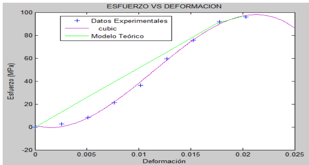
FIGURA 32 MODELACION (DIA 28 - MUESTRA 3 - 15%)
