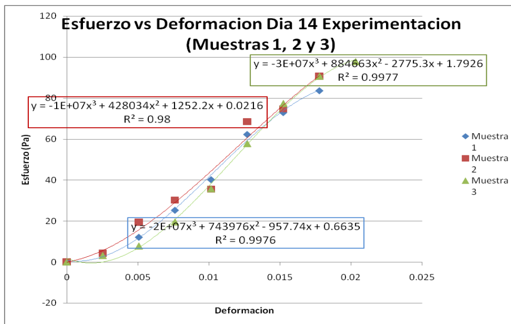
FIGURA 6 ESFUERZO VS DEFORMACION DIA14
