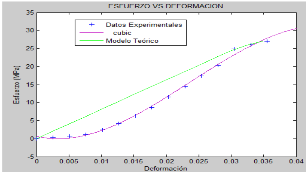
FIGURA 21 MODELACION (DIA 7 - MUESTRA 1 - 15%)
