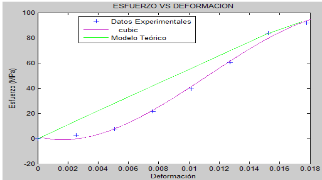
FIGURA 31 MODELACION (DIA 28 - MUESTRA 2 - 15%)
