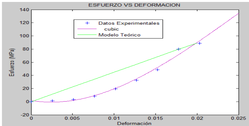
FIGURA 20 MODELACION (DIA 25 - MUESTRA 3 - 17.5%)
