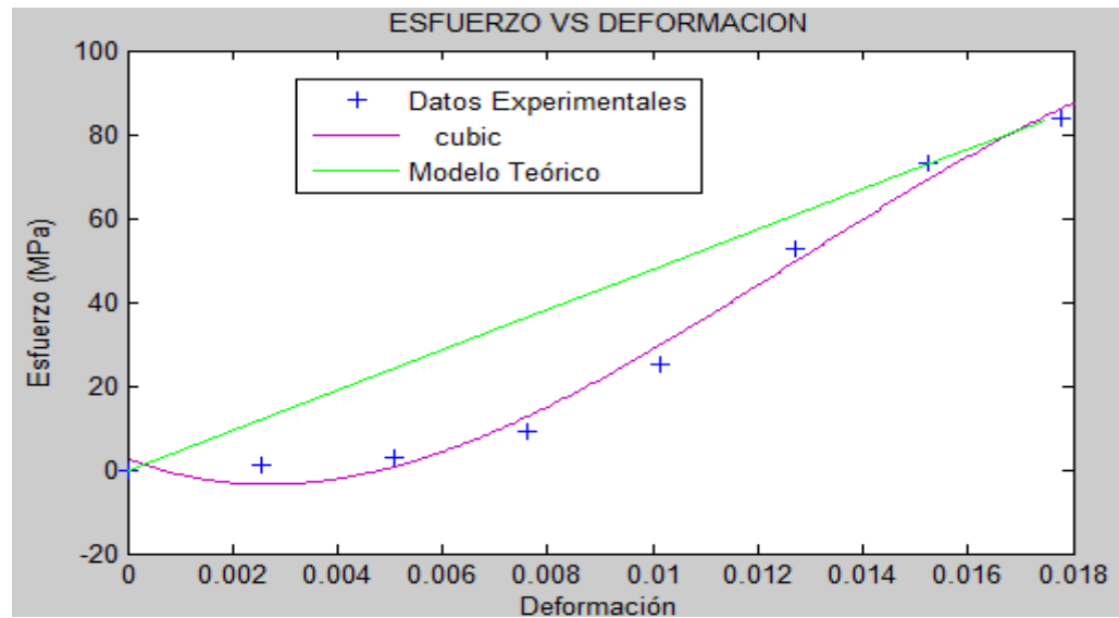
FIGURA 17 MODELACION (DIA 18 - MUESTRA 2 - 17.5%)
