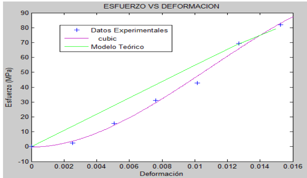
FIGURA 12 MODELACION (DIA 11 - MUESTRA 1 - 17.5%)
