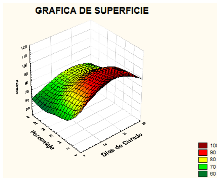
FIGURA 4.5 SUPERFICIE DE RESPUESTA (VALIDACION)
