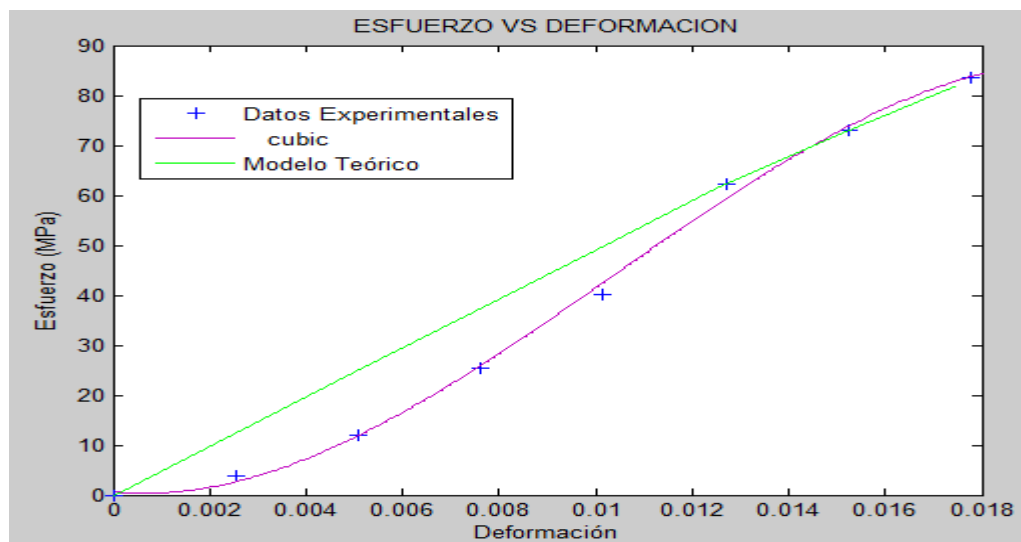
FIGURA 24 MODELACION (DIA 14 - MUESTRA 1 - 15%)
