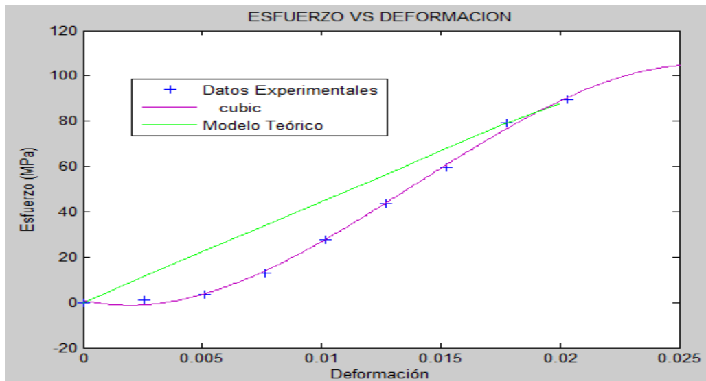
FIGURA 16 MODELACION (DIA 18 - MUESTRA 2 - 17.5%)
