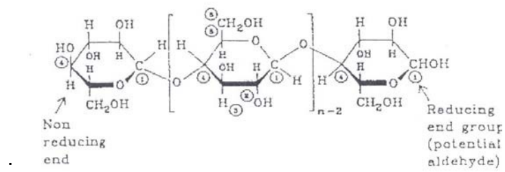
FIGURA 2.3 MOLECULA DE CELULOSA
