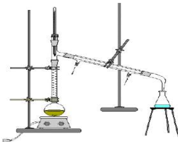
Figura 2.1 Destilación Fraccionada
