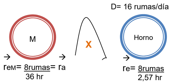
FIGURA 4.13 DATOS PARA CONWIP
