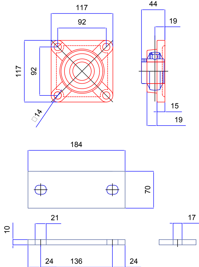
Chumacera UCF207D1
