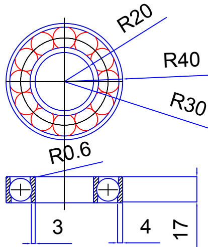
Rodamiento NTN 7008
