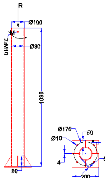
FIGURA 3.30. DIAGRAMA DEL TUBO SOPORTE DE SISTEMA DE ALIMENTACIÓN.
