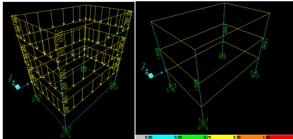
FIGURA 3.49. ANÁLISIS DE ESTRUCTURA CON PROGRAMA SAP2000.
