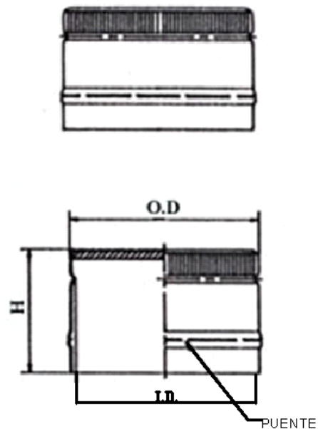
FIGURA 1.5. ESQUEMA DE TAPA INVOLABLES.
