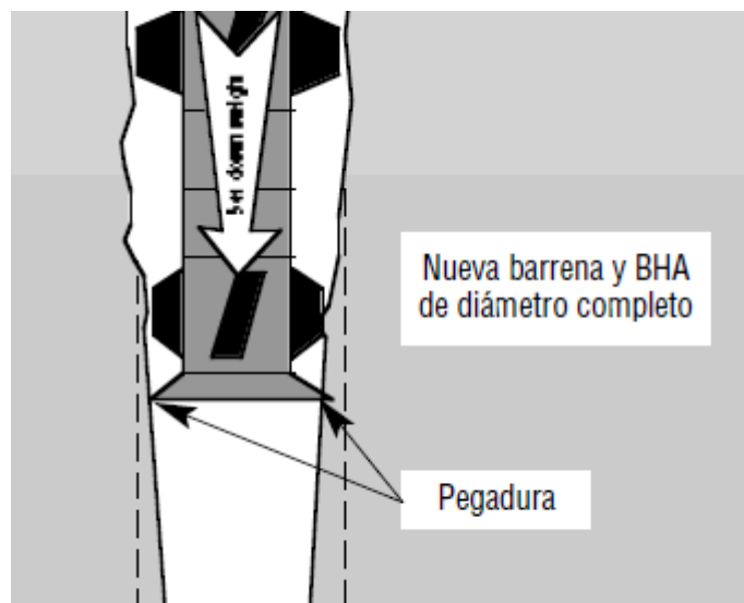
Figura 5-2. Atascamiento mecánico por diámetro reducido en el hueco. (Energy API, 2001)
