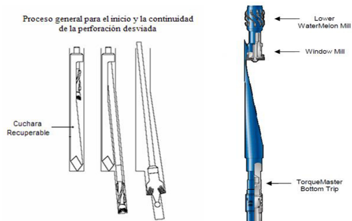
Figura 3-14. Cucharas recuperables.
