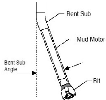
Figura 3-13. Codo desviador.
