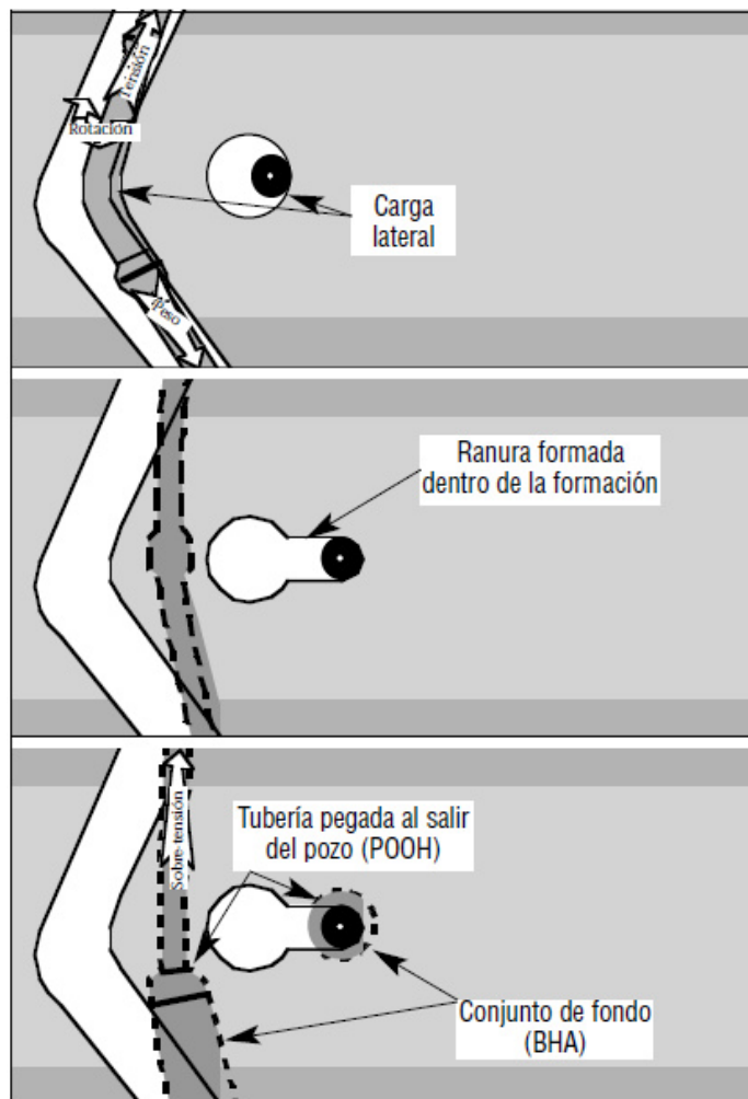
Figura 5-1. Construcción de un ojo de llave. (Energy API, 2001)
