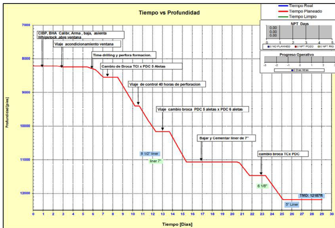
Figura 4-10. Curva de Avance del Pozo. (Elaborado por Empresa Petrolera)
