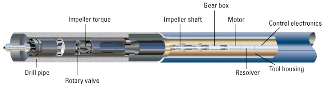
Figura 3-8. Sistema MWD Slimpulse. (Schlumberger, 2002)
