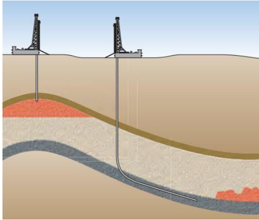
Figura 1-1. Tipos de pozo. (Schlumberger, 2011)
