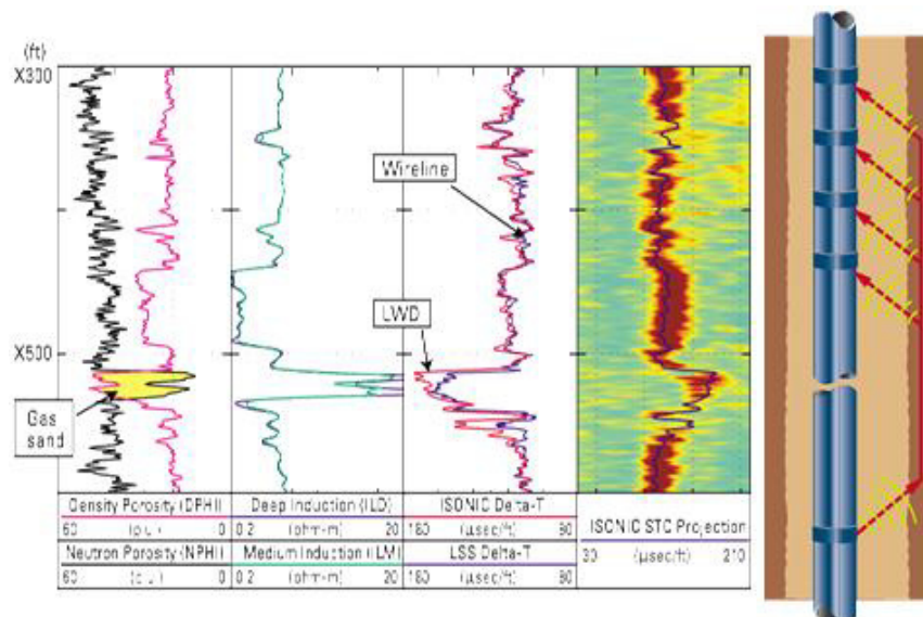
Figura 3-9. Registros eléctricos. (Elaborado por Empresa Petrolera)
