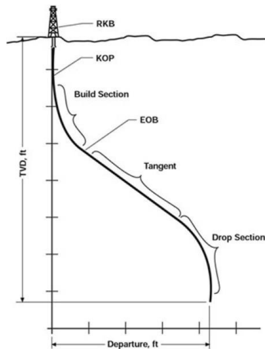
Figura 2-1. Partes de un pozo direccional. (Shoxxe, 2009)
