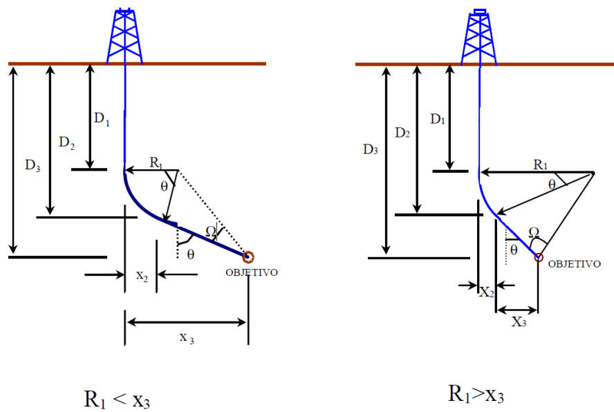
Figura 2-4. Pozo direccional tipo J (PEMEX, 2011)
