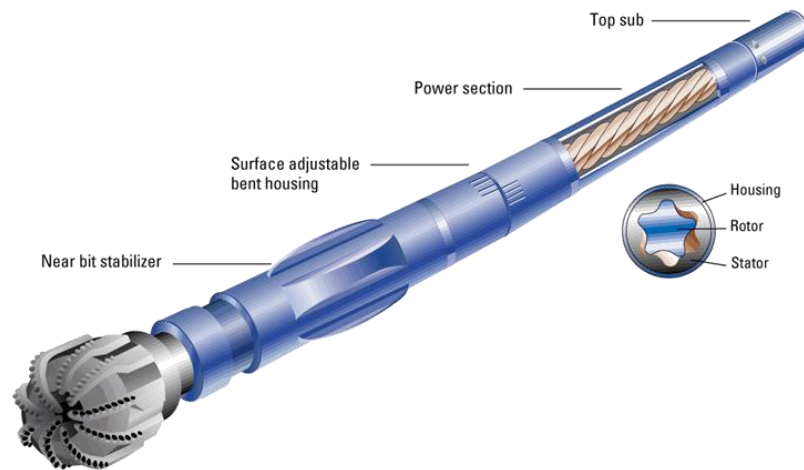
Figura 3-1. Motor de fondo PowerPak M
