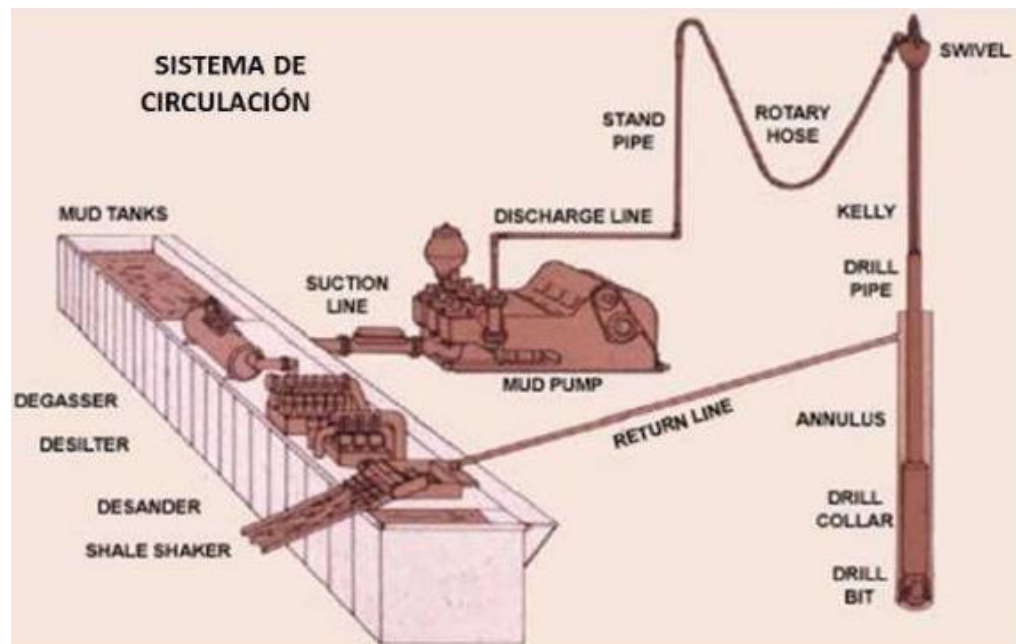
Figura 1-2. Sistema de Circulación (Aird, 2008)
