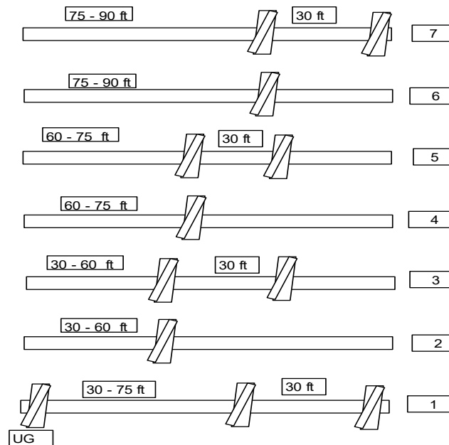
Figura 3-17. Ubicación de estabilizadores para tumbar ángulo. (Elaborado por empresa petrolera).
