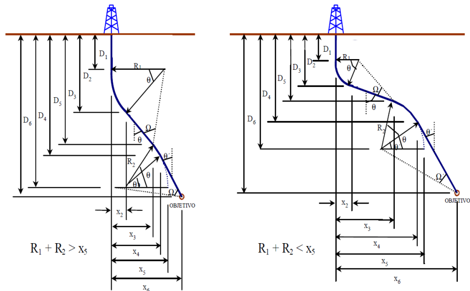
Figura 2-3. Pozo direccional tipo S modificado (PEMEX, 2011)
