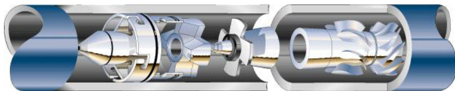
Figura 3-6. Sistema MWD Power Pulse. (Schlumberger, 2013)
