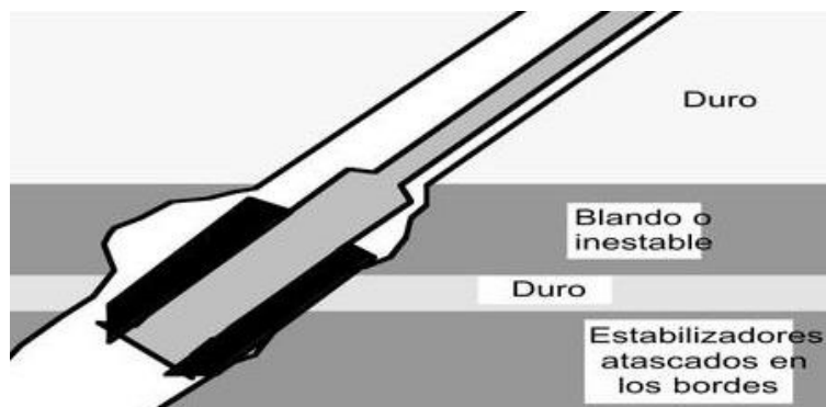
Figura 5-3. Escalones y pata de perro en el pozo. (Energy API, 2001)
