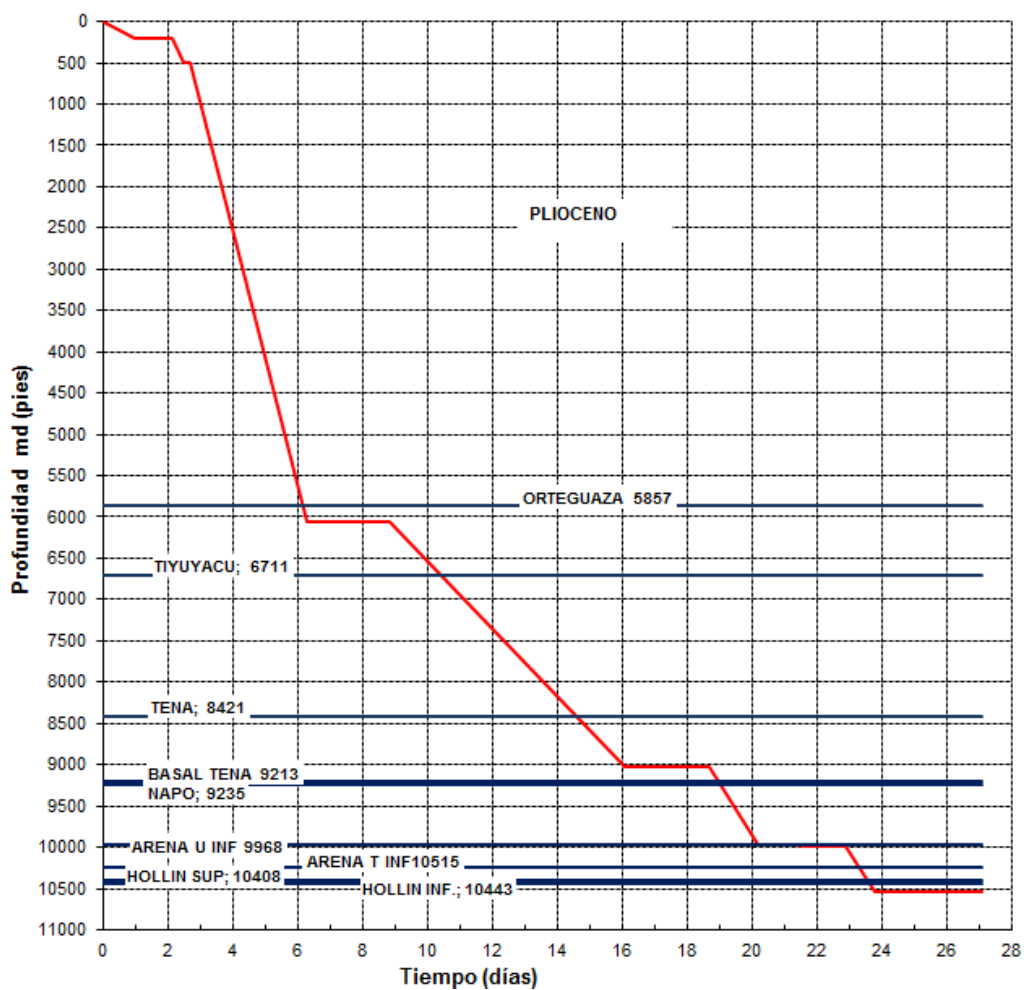
Figura 4-9. Curva de Avance del Pozo. (Elaborado por Empresa Petrolera)
