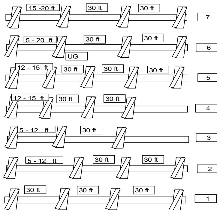
Figura 3-16. Ubicación de estabilizadores para mantener ángulo. (Elaborado por empresa petrolera).
