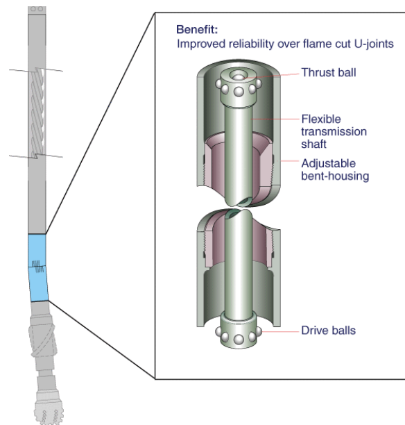
Figura 3-3. Sección ajustable. (Schlumberger, Steerable Motor Handbook , 2004)
