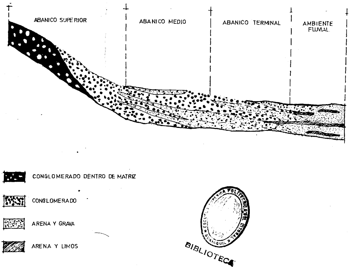
FIG. 32. LITOFACIES EN UN ABANICO ALUVIAL (8)
