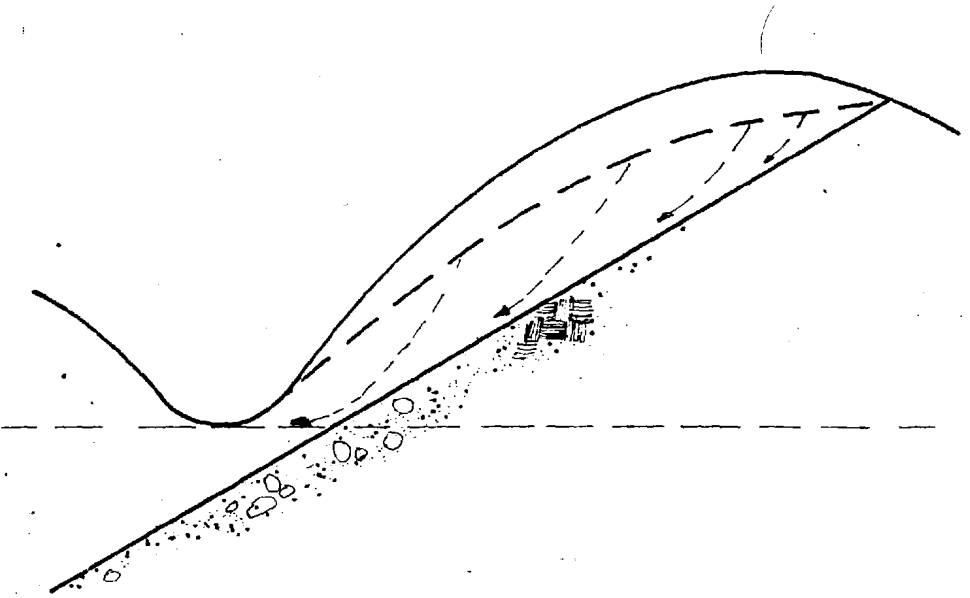
FIG.43. BASE IMPERMEABLE CERCA DE LA SUPERFICIE (1)
