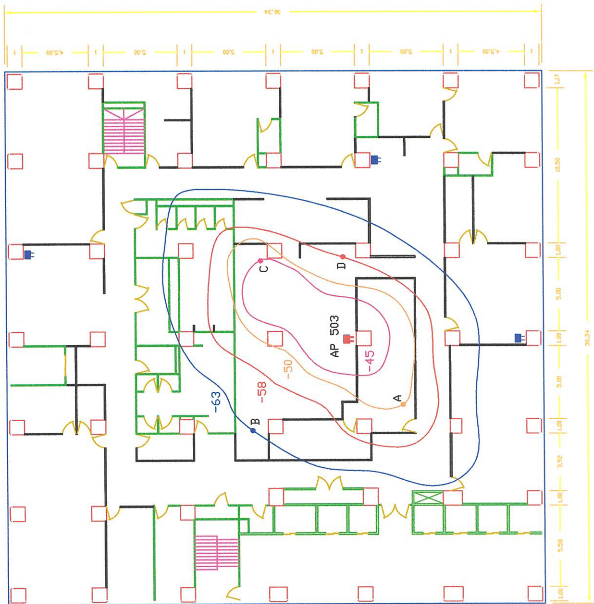
RED WI-FI DE PACIFICTEL PISO 5 - AP 503
