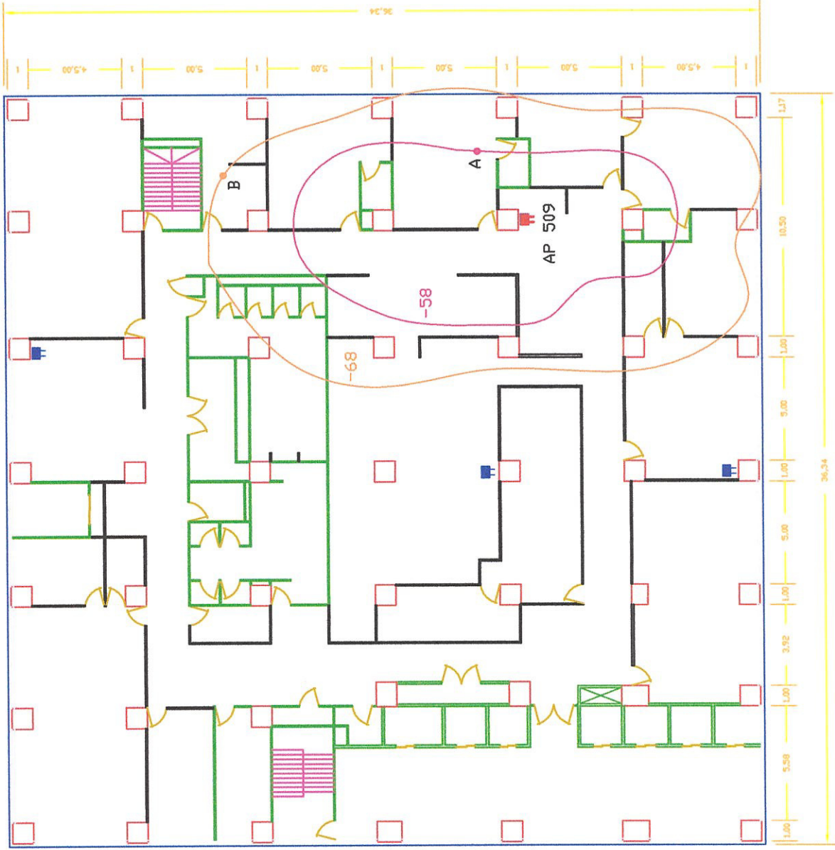
RED WI-FI DE PACIFICTEL PISO 5 - AP 509
