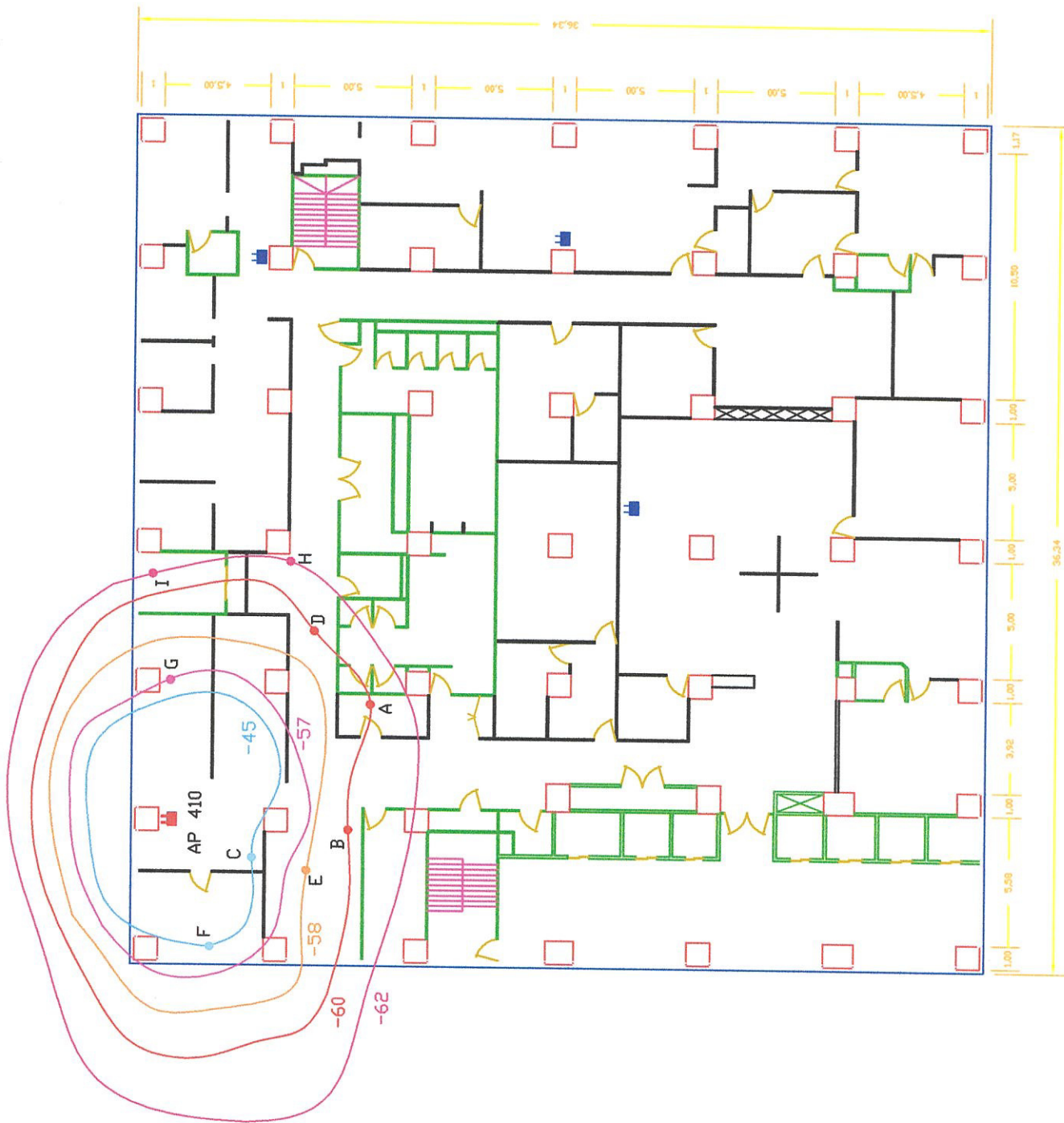
RED WI-FI DE PACIFICTEL PISO 4 - AP 410
