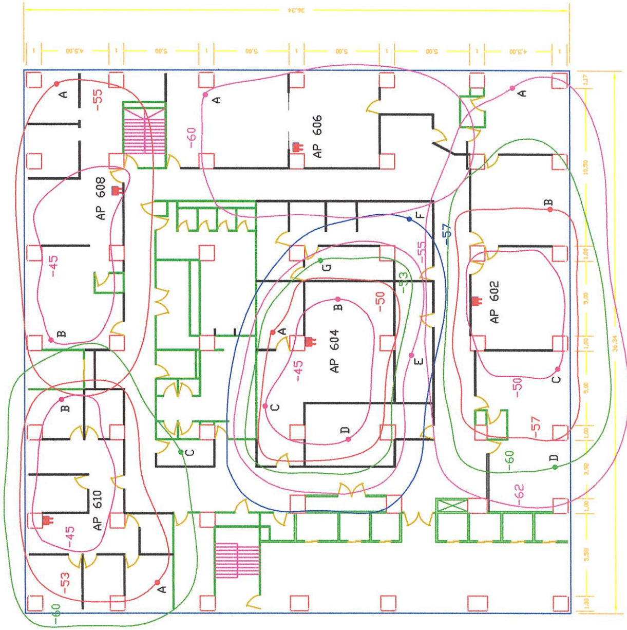
RED WI-FI DE PACIFICTEL PISO 6
