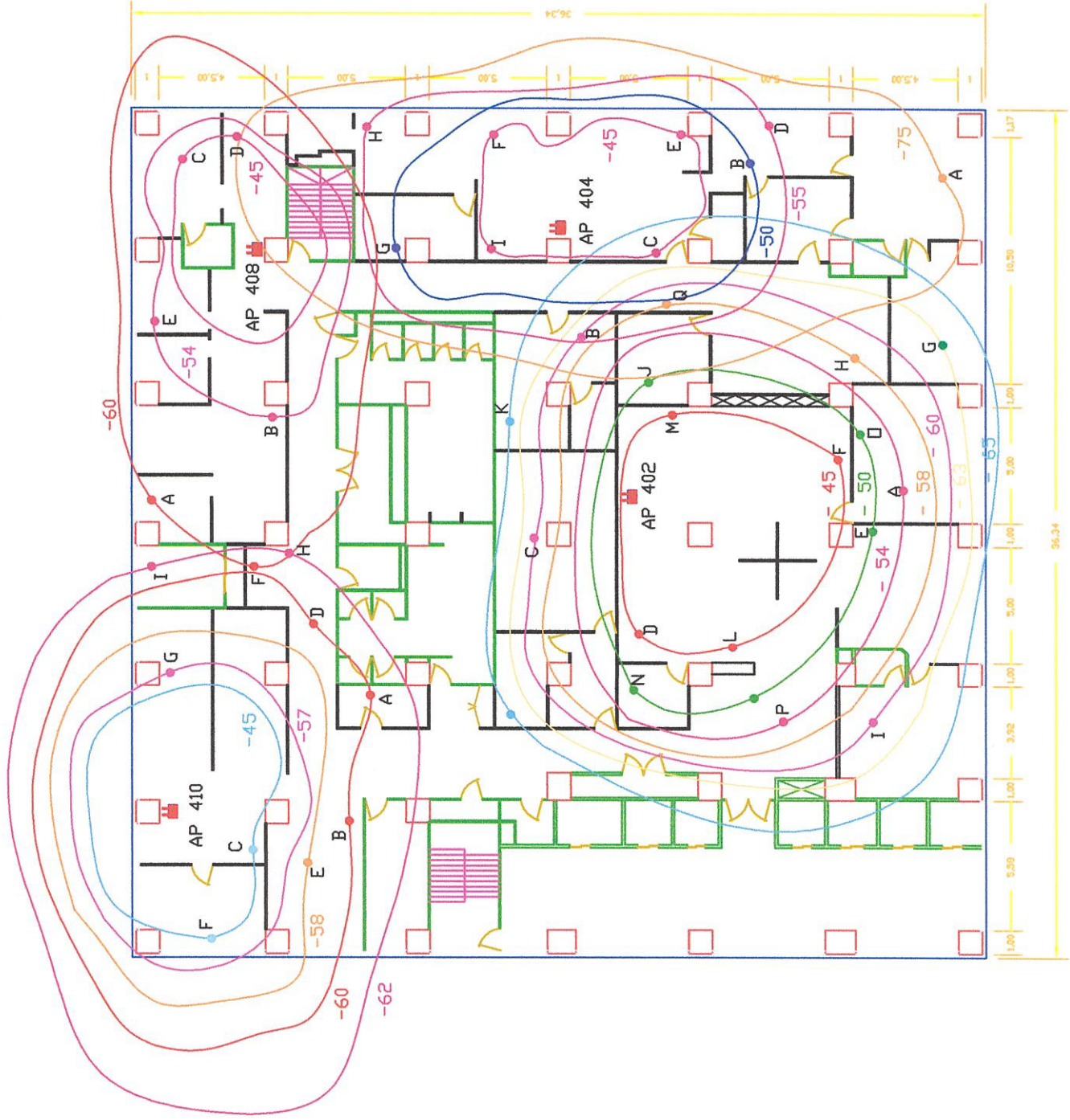
RED WI-FI DE PACIFITEL PISO 4
