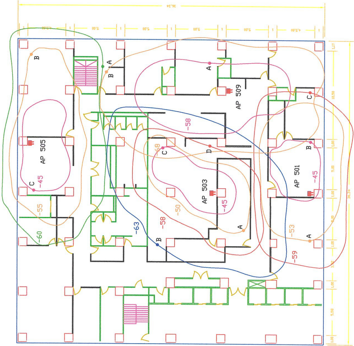
RED WI-FI DE PACIFICTEL PISO 5
