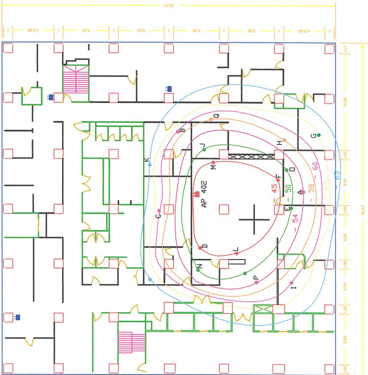
RED WI-FI DE PACIFICTEL PISO 4 - AP 402
