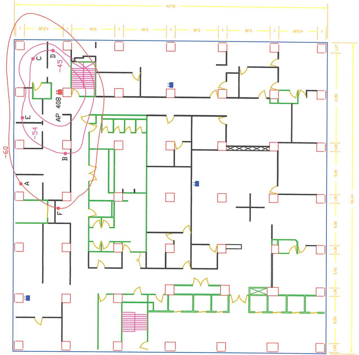
RED WI-FI DE PACIFICTEL PISO 4 - AP 408
