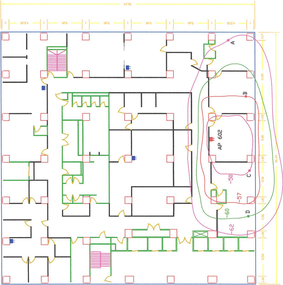
RED WI-FI DE PACIFICTEL PISO 6 - AP 602
