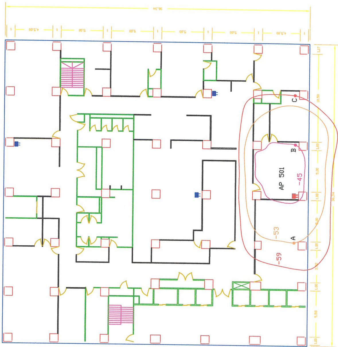
RED WI-FI DE PACIFICTEL PISO 5 - AP 501
