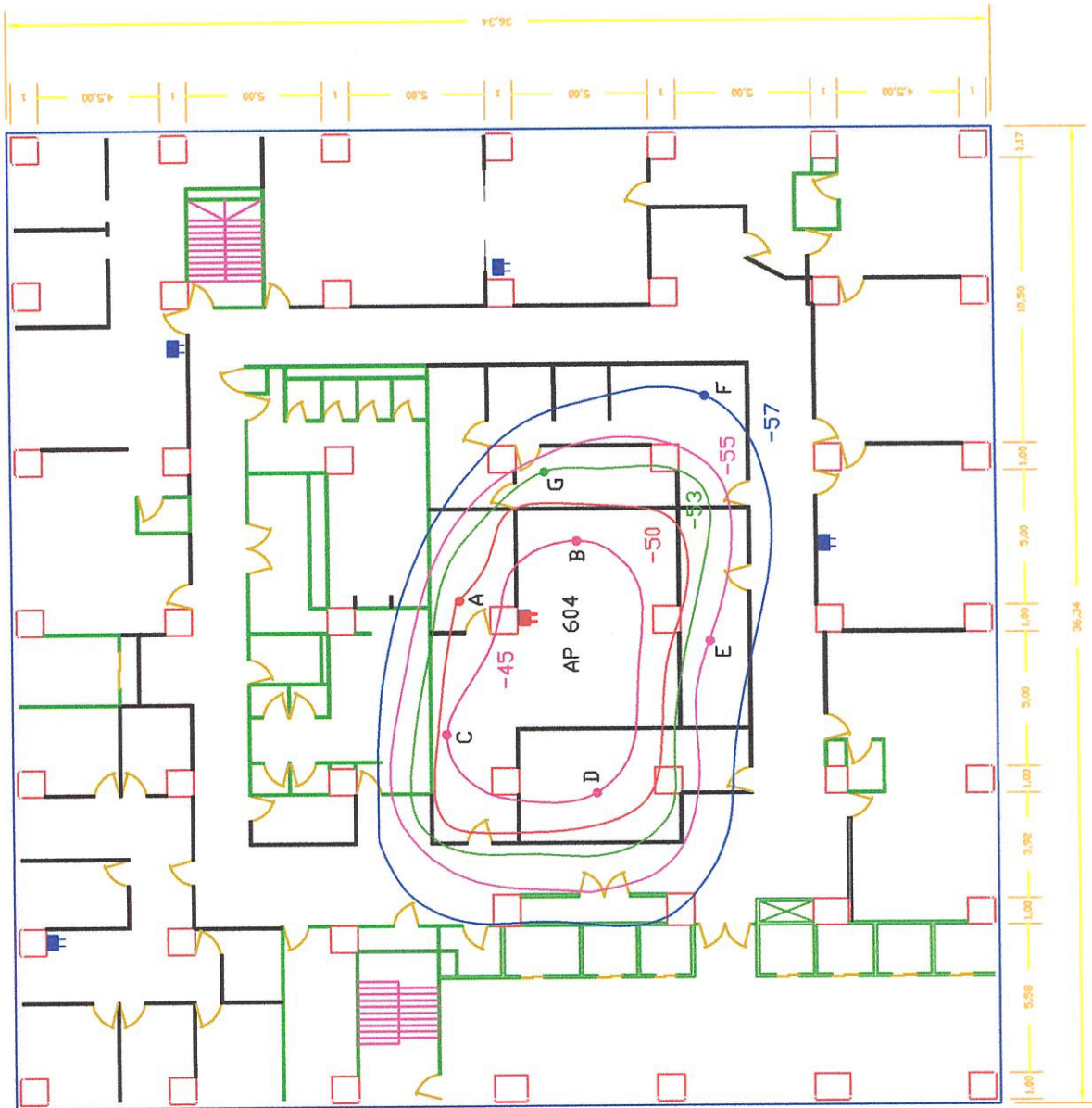
RED WI-FI DE PACIFICTEL PISO 6 - AP 604
