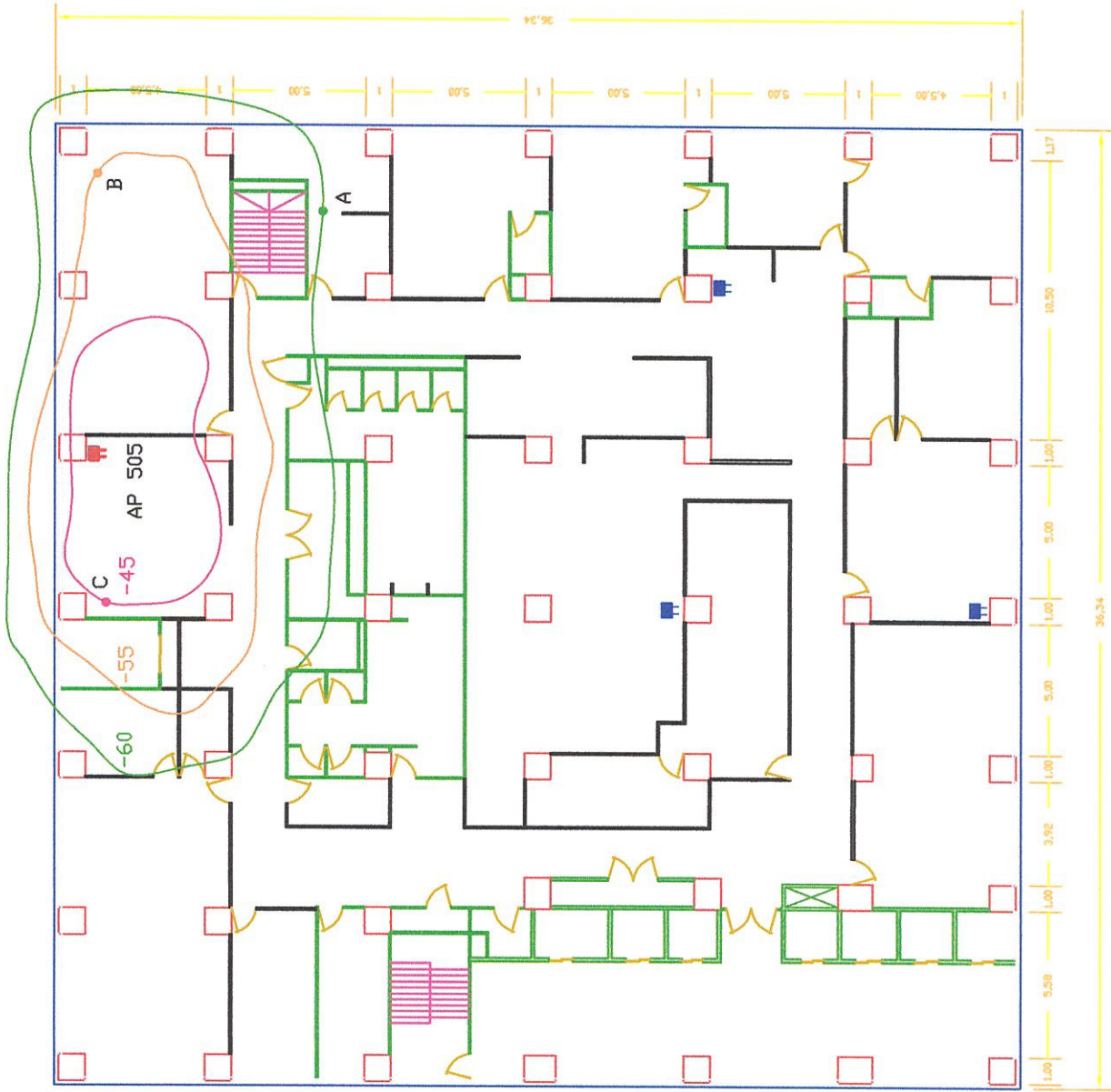
RED WI-FI DE PACIFICTEL PISO 5 - AP 505
