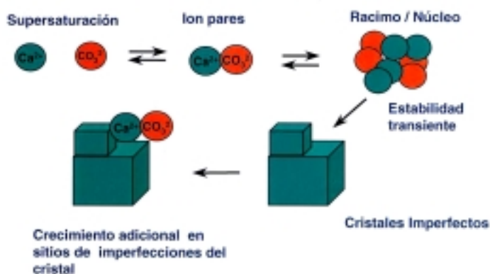
FIG. 1.7 Mecanismo de precipitación de la incrustación
