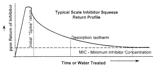
Fig 4.2 Perfil de Retorno de un tratamiento típico de Inhibidor de incrustaciones.
