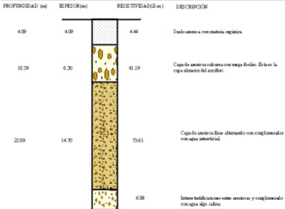
Ajuste matemático y columna geoelectrica del A-05 correspondiente a la Hacienda ESPOL-PECHICHE
