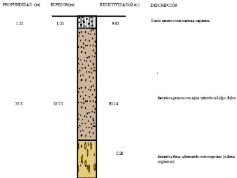
Ajuste matemático y columna geoelectrica del M-02 correspondiente al Museo Real
