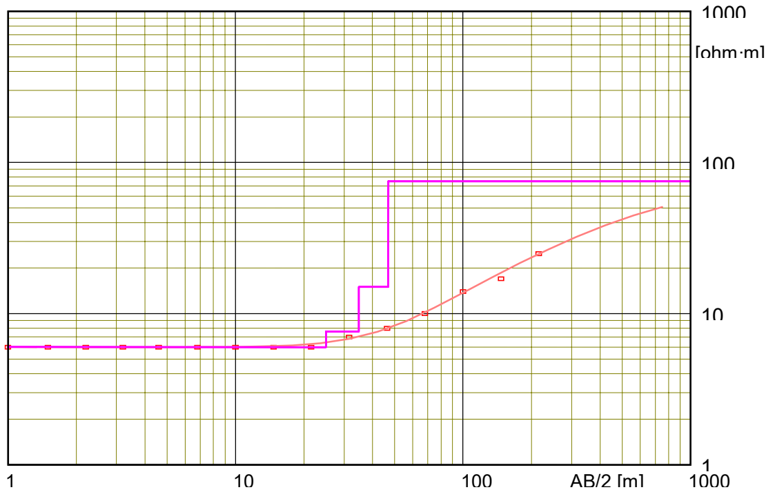
Columna Geoeléctrica del Sondeo A6
