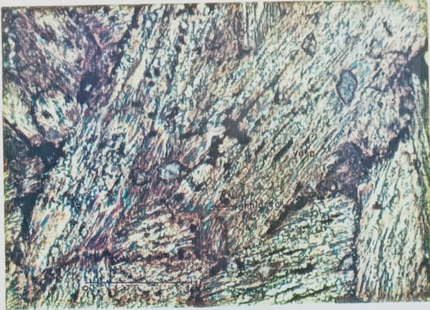
Lámina 1126 - Objetivo 6.3x - Nícoles cruzados. Yeso con pequeña alteración a anhidrita en los bordes.
