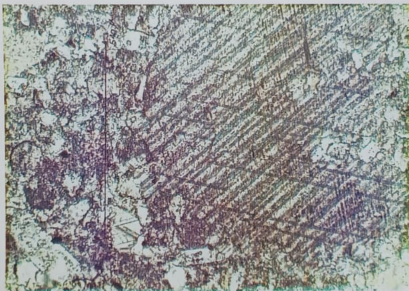
Lámina 1129—Objetivo 6.3x — Nícoles paralelos. Vista panorámica de esparita (cavidad), con macla lamelar y clivaje romboédrico.
