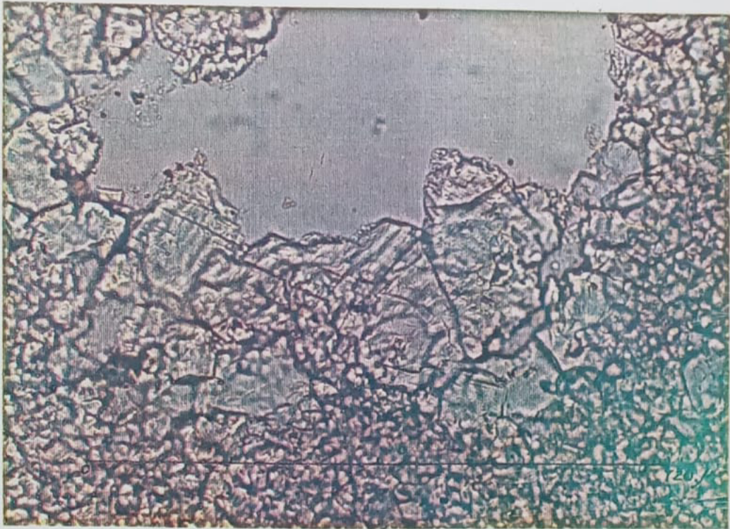
Lámina 1130—Objetivo 25 x — Nícoles paralelos. Se observa detalle de una cavidad de desmicritización.
