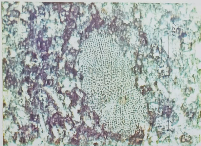
Lámina 1128—Objetivo 6.3x — Nícoles paralelos. Vista panorámica con estructura fósil (Briozoos).
