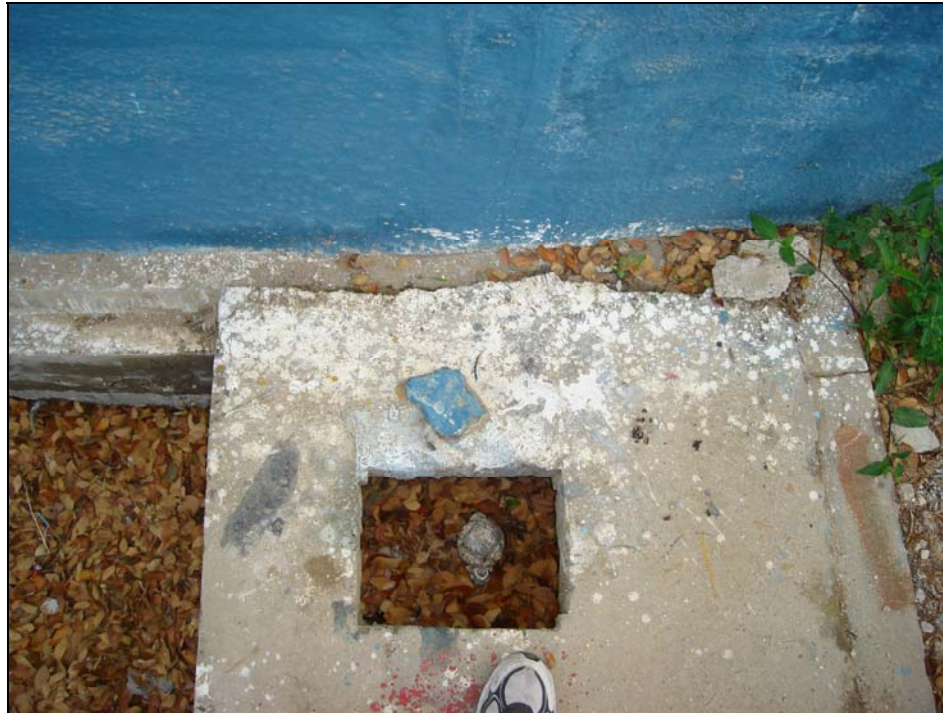
Figura. 3.6 VALVULA DE APERTURA PARA RECEPCION DE AGUA DEL CIRCUITO SUBMARINO (MAR-TIERRA)
