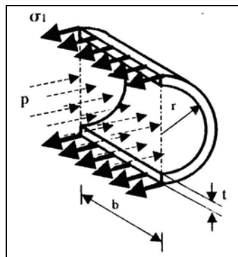
Figura 1.3 ESFUERZO CIRCUNFERENCIAL
