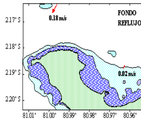
Figura. 2.8 VELOC. CORRIENTE
