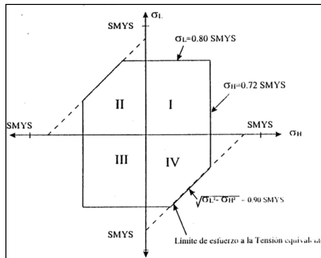
Figura. 1.4 ESFUERZOS PERMISIBLES ANSI B31.4
