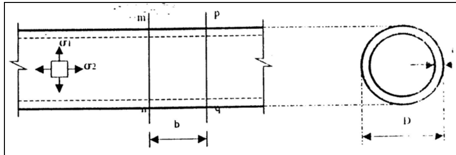
Figura 1.1 CORTE DE UNA TUBERÍA
