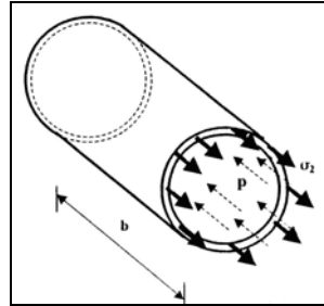
Figura 1.2 ESFUERZO LONGITUDINAL
