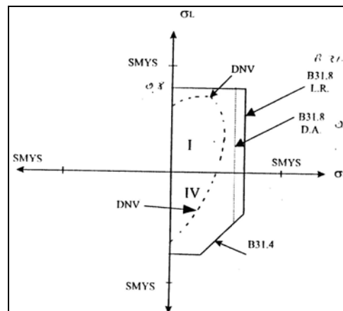
Figura. 1.9 DNV (OPERACIONAL Y AMBIENTAL) CONTRA B31.4 Y B31.8
