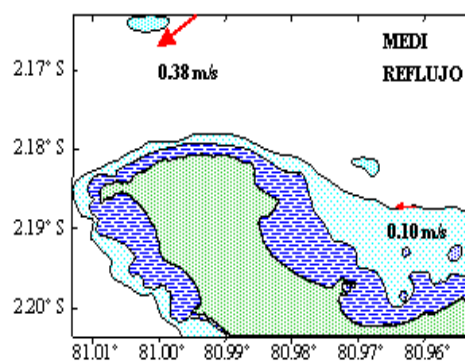
Figura. 2.6 VELOC. CORRIENTE
