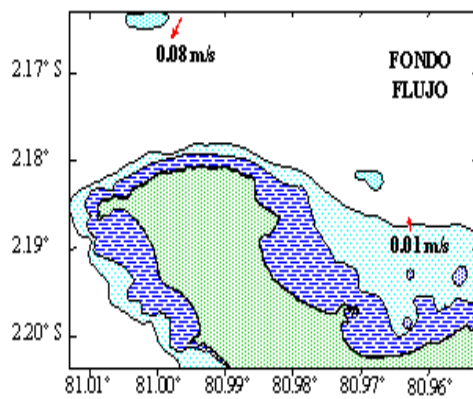
Figura. 2.7 VELOC. CORRIENTE
