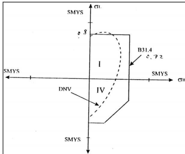
Figura. 1.8 DNV (OPERACIONAL) CONTRA B31.4 (PRESIÓN Y CARGA)
