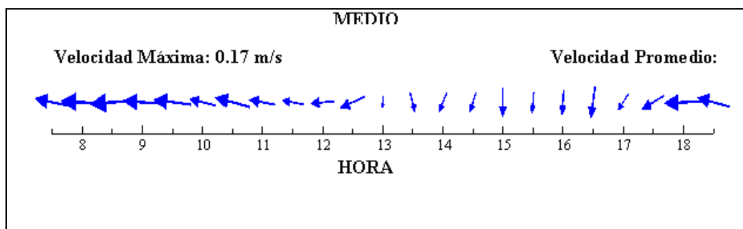
Figura. 2.10 PERFILES DE VELOCIDAD MAXIMO Y PROMEDIO OBTENIDOS ESTACION 1 (MEDIO)
