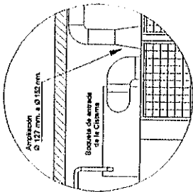
DETALLE A - A
