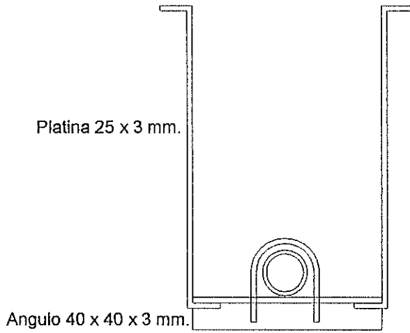
Soporte de tubería en el aire
