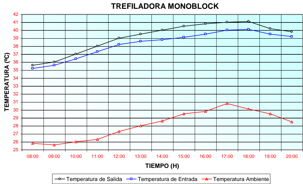
Figura 2.16 Temperatura del agua de enfriamiento (Tref. Monoblock)
