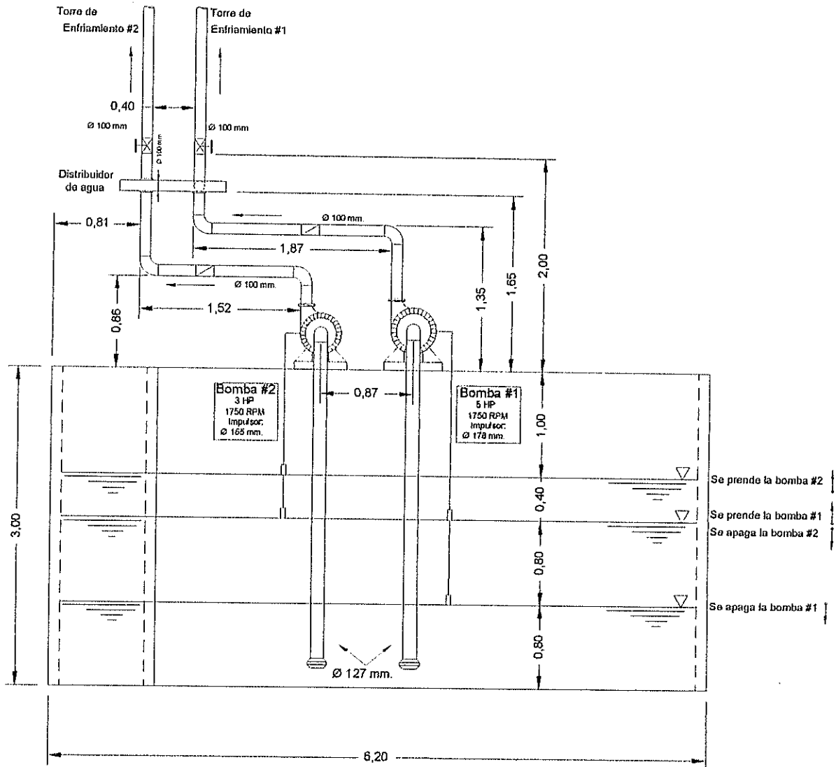
CISTERNA INTERNA DE LA PLANTA
