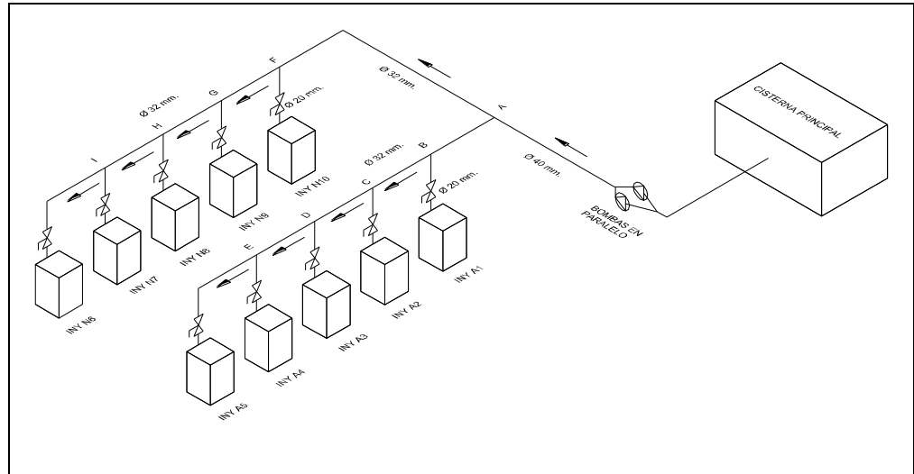
Figura 4.11 Distribución de tuberías (inyectoras)
