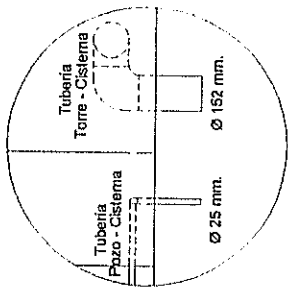
DETALLE B - B
