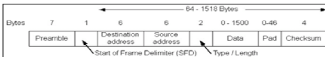
Figura 1.12 Trama Ethernet 64-1518 bytes
