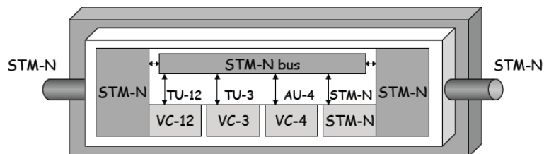
Figura 1.4 Equipo Regenerador [11]
