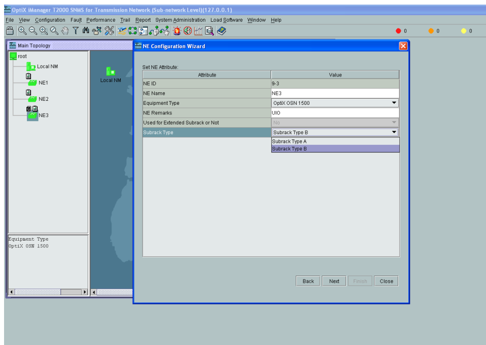
Figura 3.9 Tipo de subrack del Optix OSN 1500B
