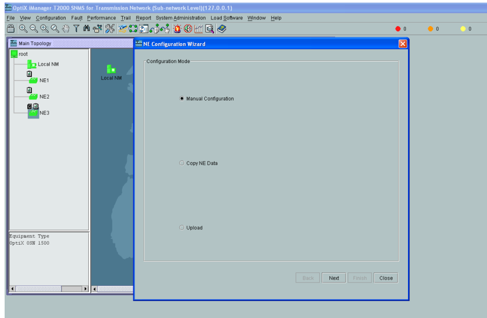
Figura 3.8 Configuración Manual
