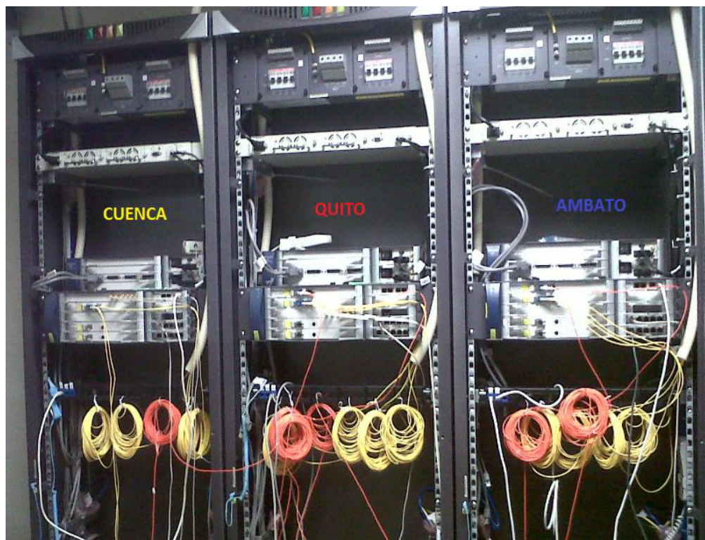
Figura 3.2 Conexiones de los equipos Huawei (Optix OSN 1500)
