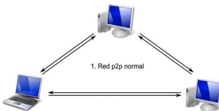
Figura 2.4: Sistema P2P [15]
