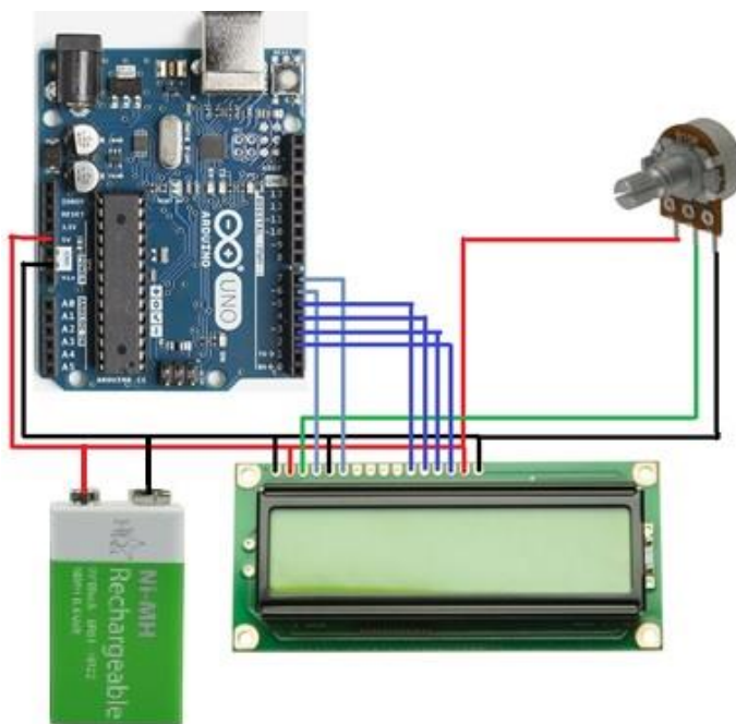
Figura 3.23 Diagrama de conexión del módulo en parada
