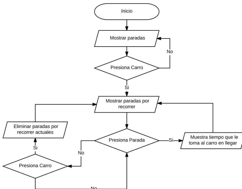
Figura 3.19 Algoritmo de interacción entre el usuario y la interfaz web para conocer las paradas que faltan por recorrer a un vehículo seleccionado
