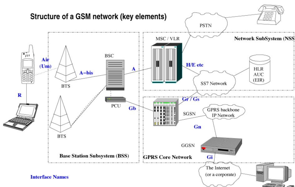
Figura 2.5 Arquitectura de una red GSM [23]
