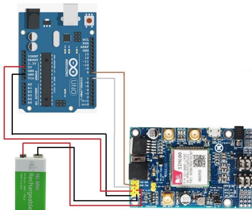
Figura 3.2 Diagrama de conexión del módulo en vehículo
