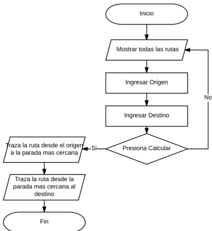
Figura 3.22 Algoritmo que representa la interacción entre el usuario y la opción de calcular ruta
