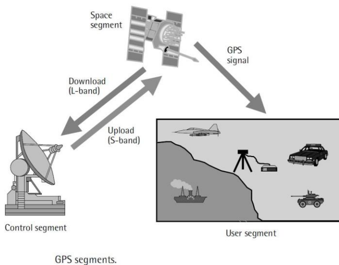
Figura 2.6 Red GPS utilizada para la obtención de las coordenadas y velocidad del móvil [25]
