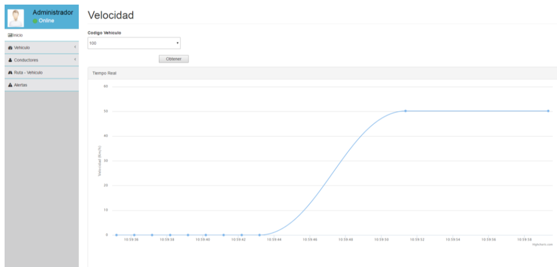
Figura B 5 Pantalla que muestra gráfico de velocidad en tiempo real por cada vehículo
