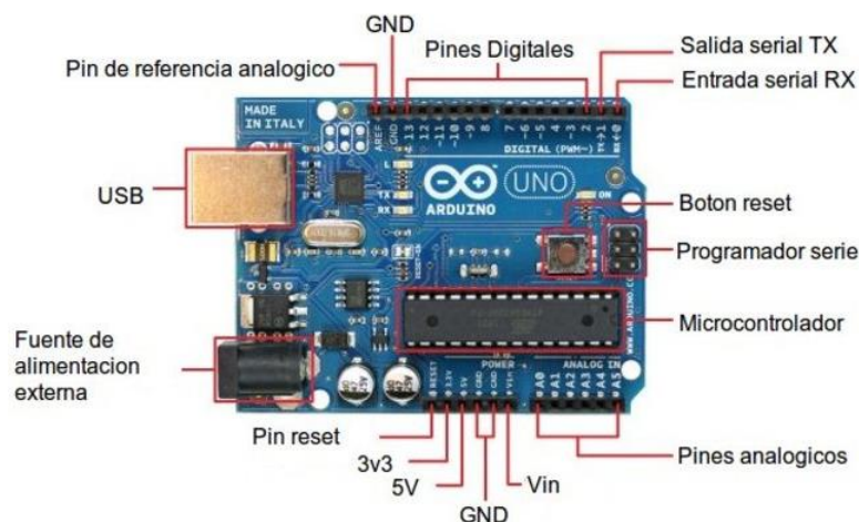
Figura 2.1 Placa electrónica Arduino UNO, Empleada para la interconexión de los dispositivos [16]
