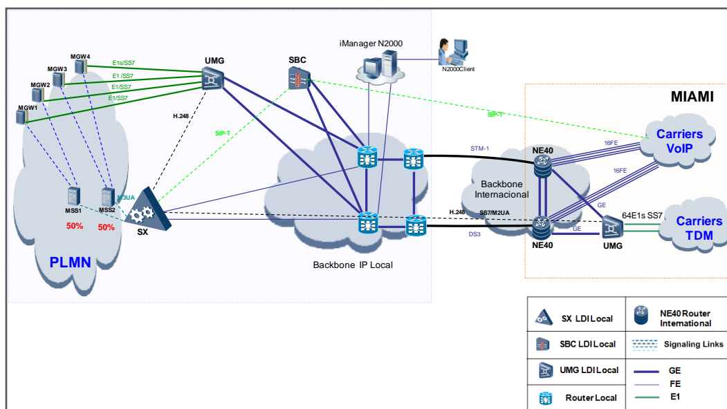
Figura 1.2: Topología Estándar de una red LDI local
