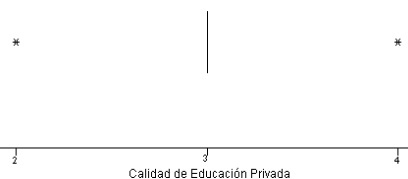
Diagrama de Caja
