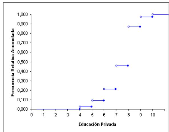
Gráfico de la Distribución Empírica
