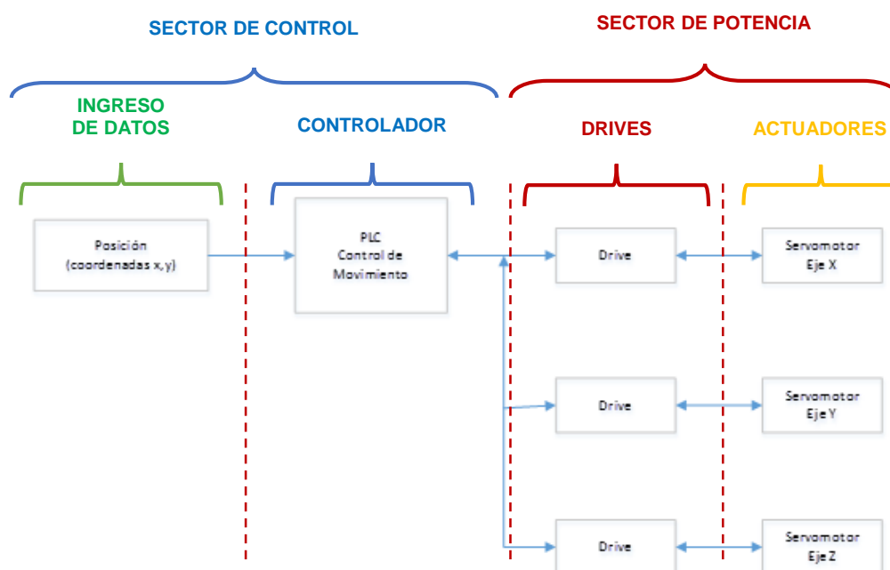
Figura 2.16: Diagrama de flujo del sector de Control y Potencia.
