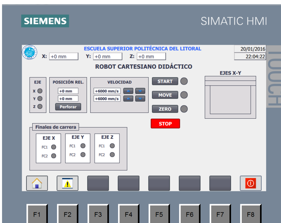
Figura 3.6: Pantalla principal del HMI.
