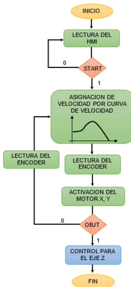
Figura 2.4: Diagrama de bloques del Controlador para eje X, Y en lazo cerrado.
