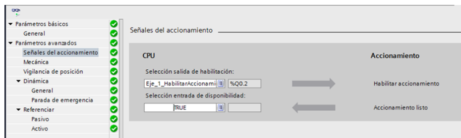
Figura 2.10: Configuración objeto tecnológico EJE: Parámetros avanzados – Señales de accionamiento.
