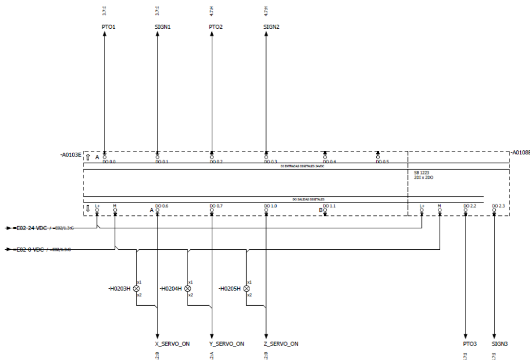
Figura 3.5: Plano de distribución 2 de entradas y salidas del PLC.
