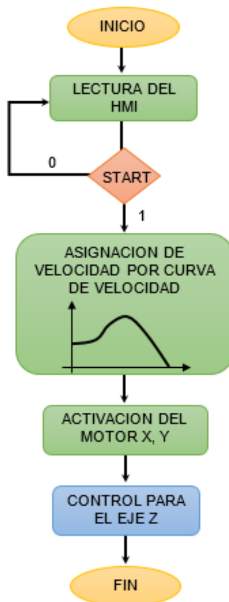
Figura 2.5: Diagrama de bloques del Controlador para eje X, Y en lazo abierto.
