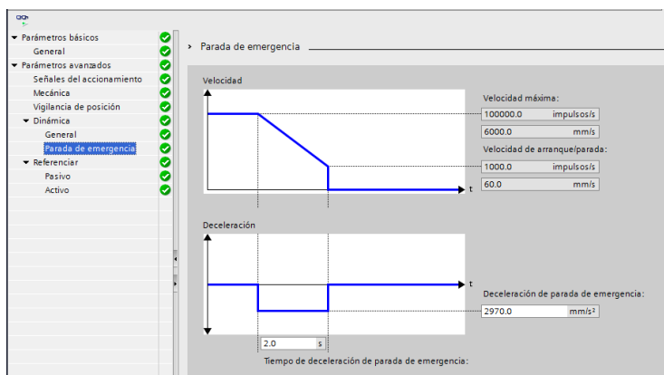
Figura 2.14: Configuración objeto tecnológico EJE: Parámetros avanzados – Dinámica – Parada de emergencia.
