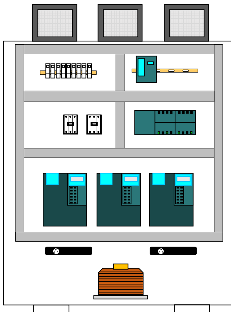
Figura 3.1: Esquema interno del Panel Eléctrico.
