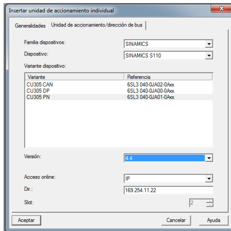
Figura 1: Insertar nuevo accionamiento
