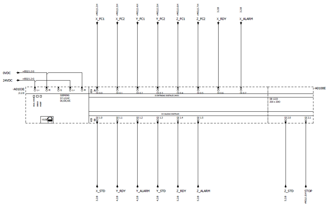
Figura 3.4: Plano de distribución 1 de entradas y salidas del PLC.
