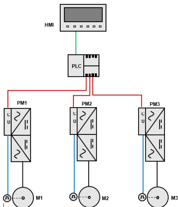
Figura 2.17: Esquema general del robot con sus elementos de potencia y de control.
