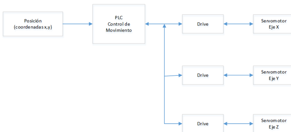
Figura 2.2: Diagrama de flujo del funcionamiento del robot cartesiano.
