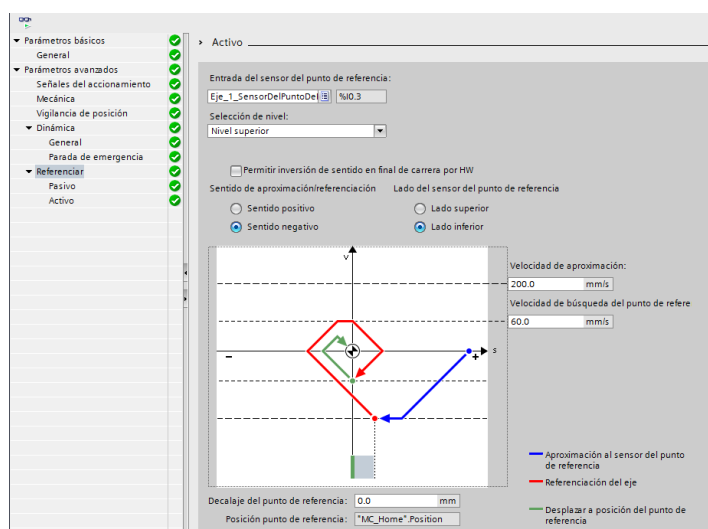
Figura 2.15: Configuración objeto tecnológico EJE: Parámetros avanzados – Referenciar.
