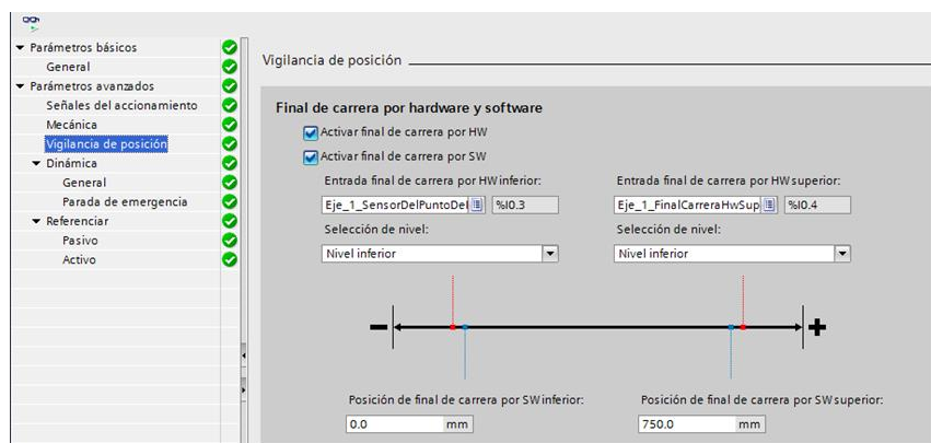
Figura 2.12: Configuración objeto tecnológico EJE: Parámetros avanzados – Vigilancia de posición.
