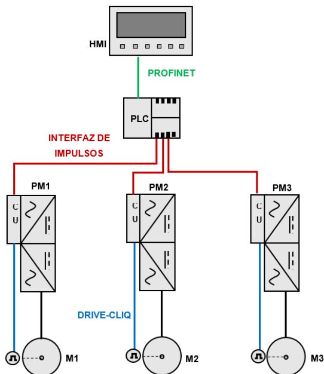
Figura 2.3: Esquema general del sector de control y sus comunicaciones.
