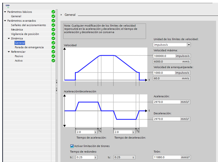
Figura 2.13: Configuración objeto tecnológico EJE: Parámetros avanzados – Dinámica – General.
