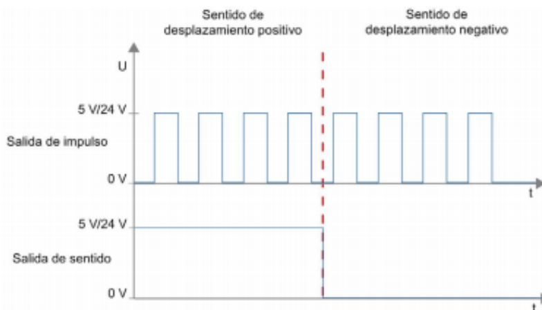
Figura 2.7: Salida de Tren de Pulsos y Sentido de giro [3].
