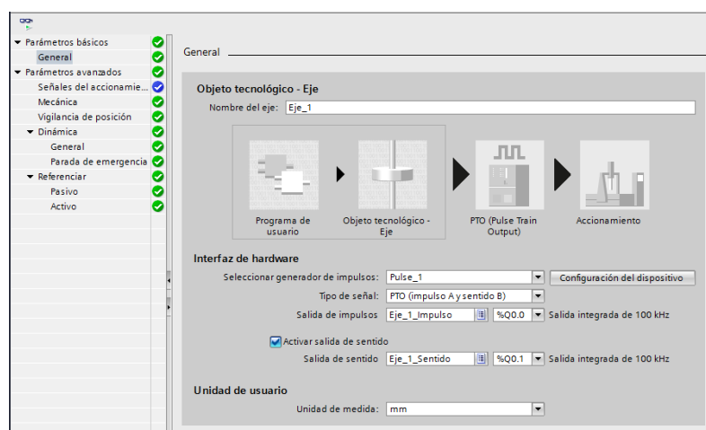
Figura 2.9: Configuración objeto tecnológico EJE: Parámetros básicos.
