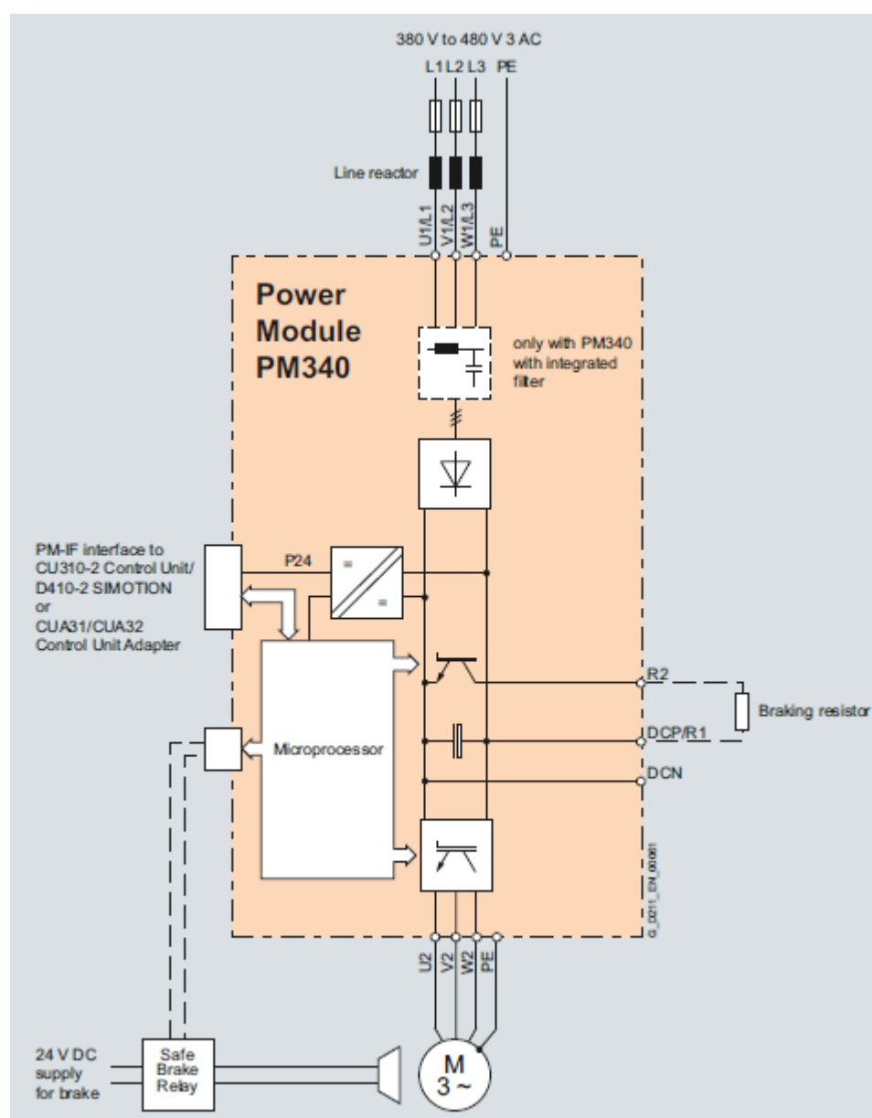
Figura 2.21: Esquema del Power Module [9].
