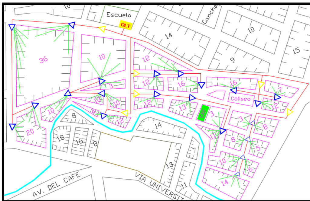
Figura 3.6: Colocación y distribución de Splitters.
