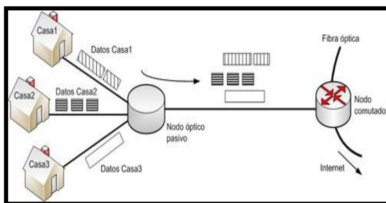
Figura 2.6: Red Pasiva punto multipunto [16].
