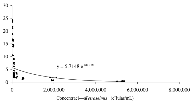
Figura 6: Respuesta de la tasa de aclaramiento de B. rotundiformis a la concentración de Tetraselmis sp. a 24°C (a), 28°C (b) y 32°C (c).
