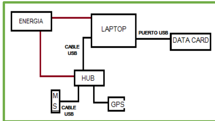
Figura 2.14: Diagrama de Conexiones de equipos para DT
