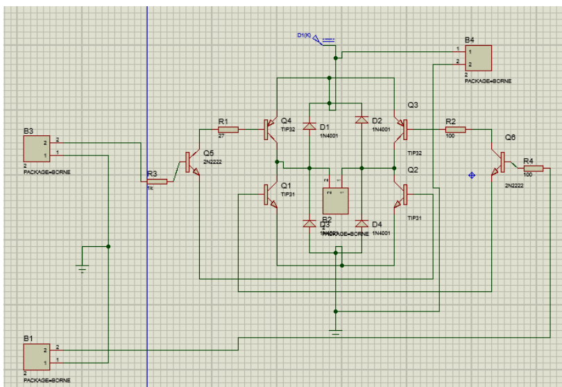
Figura 3.19: Esquemático del Puentes H.
