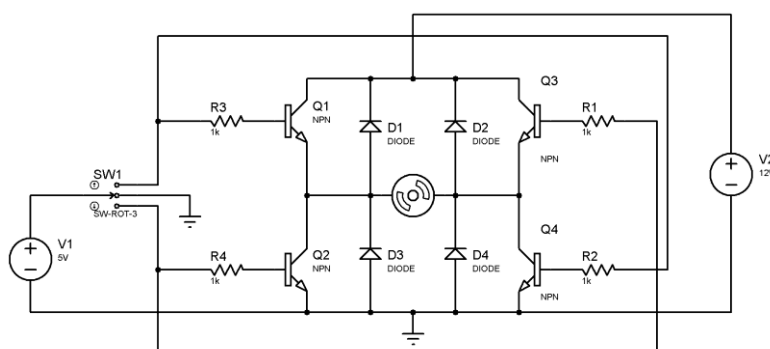
Figura 2.5: Puente H.
