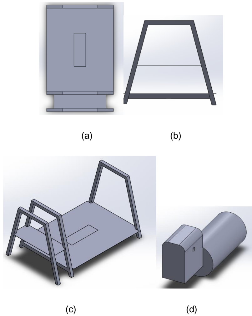
Figura 3.3: a) Bases para la Batería y el Motor DC, b) Soporte de la Base, c) Base Final, d) Motor DC.
