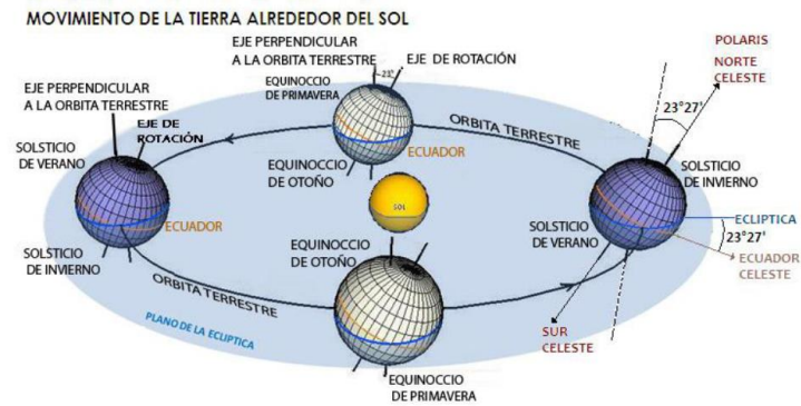
Figura 2.1: Trayectoria Sol-Tierra.
