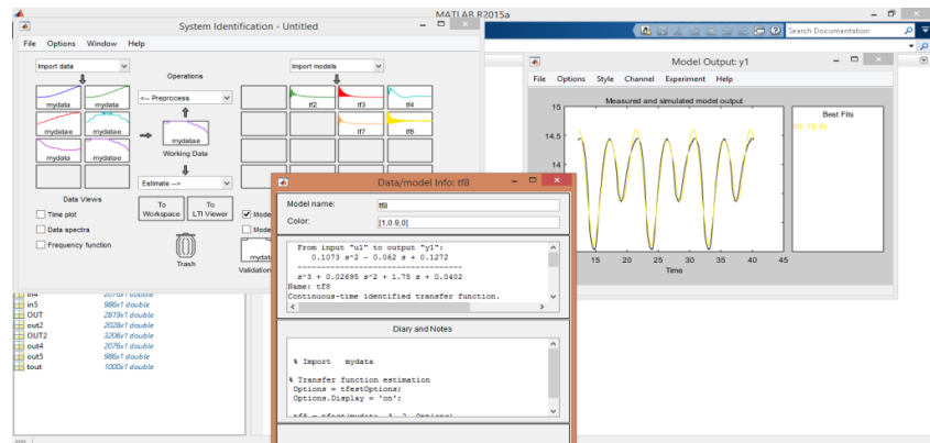
Figura 3.35: Función Transformada.
