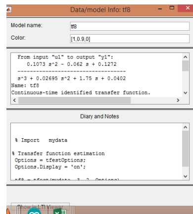
Figura 3.36: Obtención de Función de Transferencia.
