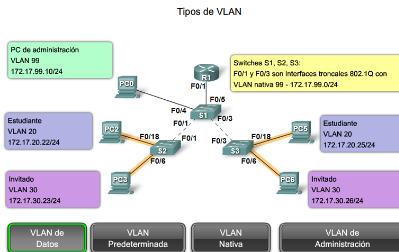
Figura 3.14: Tipos de VLAN
