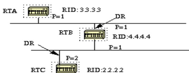
Figura 3.9: Adyacencia: Elección DR.
