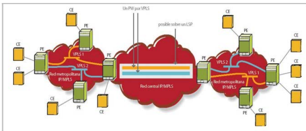
Figura 3.36: H- VPLS Usado como servicio intermetropolitano
