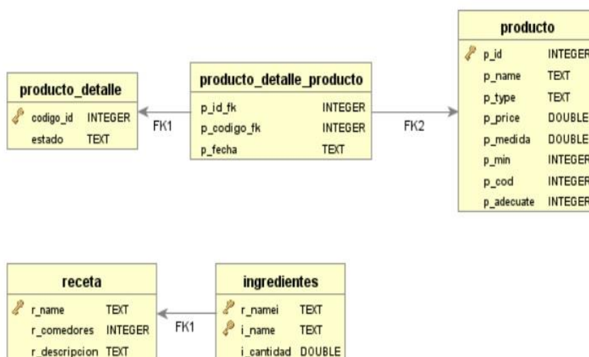
Figura 3.1: Modelo lógico de la base de datos.
