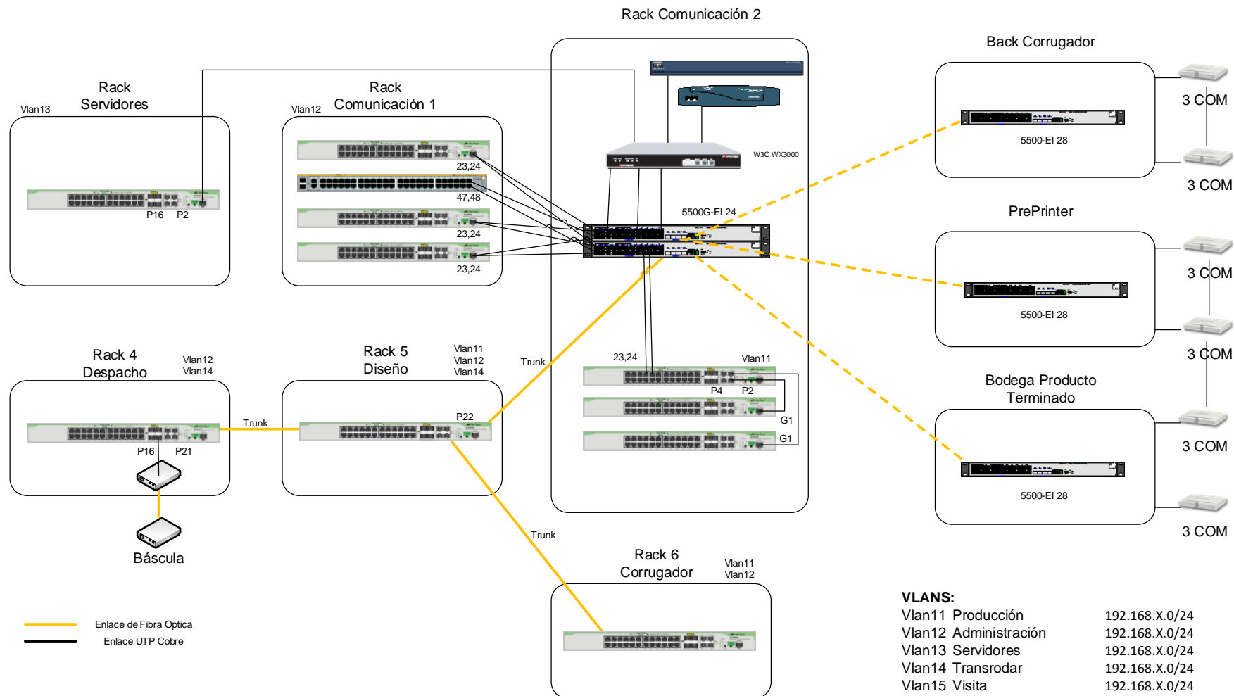
Figura 1.2: Diseño Físico de Red Actual
