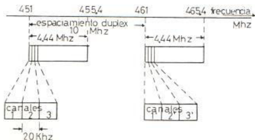
FIGURA 46.- BANDAS DE FRECUENCIA APROVECHABLES
