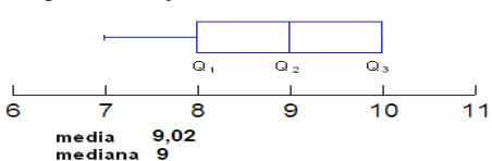
Diagrama de Caja sin valores aberrantes
