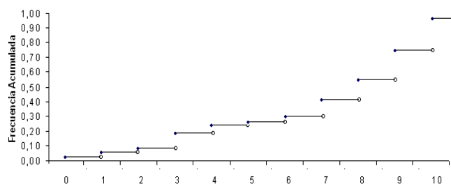
Distribución Empírica
