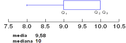
Diagrama de Caja sin valores aberrantes
