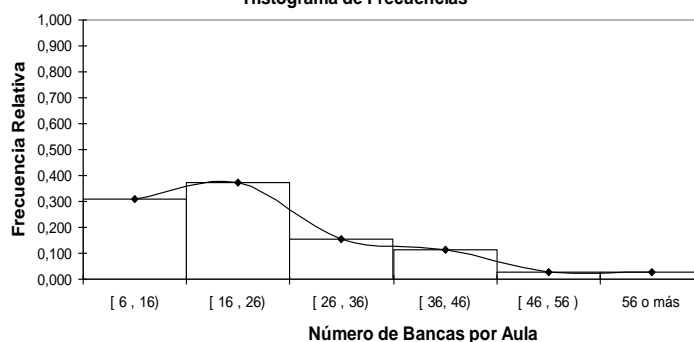
Histograma de Frecuencias
