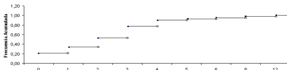
Distribución Empírica
