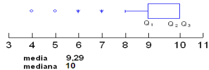
Diagrama de Caja con valores aberrantes
