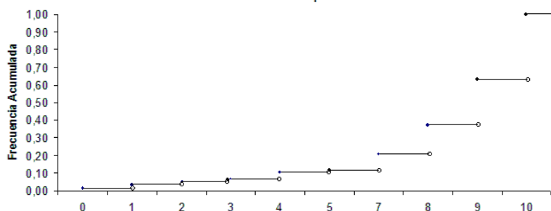
Distribución Empírica
