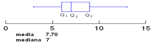
Diagrama de Caja sin valores aberrantes
