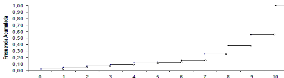
Distribución Empírica
