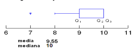
Diagrama de Caja con valores aberrantes
