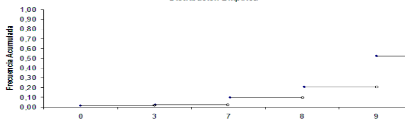
Distribución Empírica
