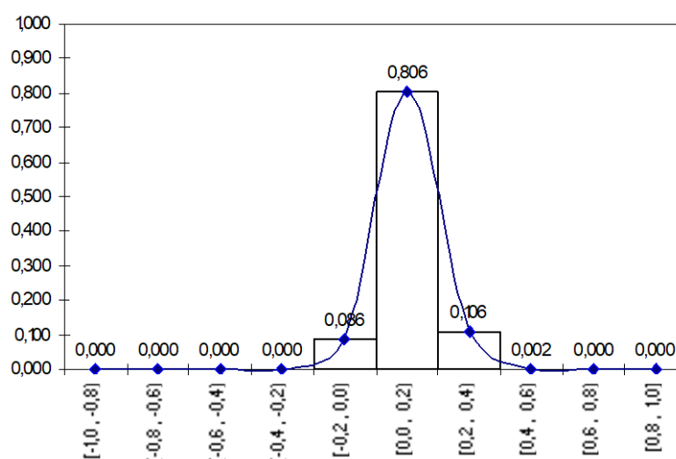
Histograma de los Coeficientes de Correlación
