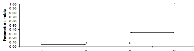
Distribución Empírica
