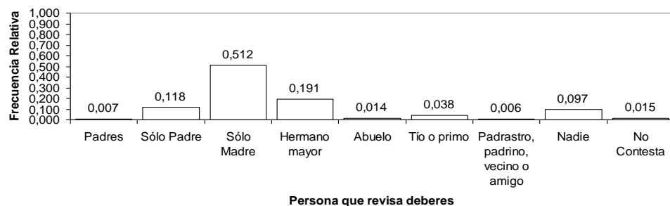
Histograma de Frecuencias
