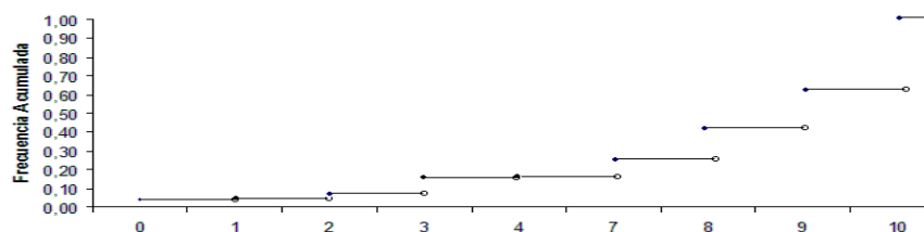
Distribución Empírica
