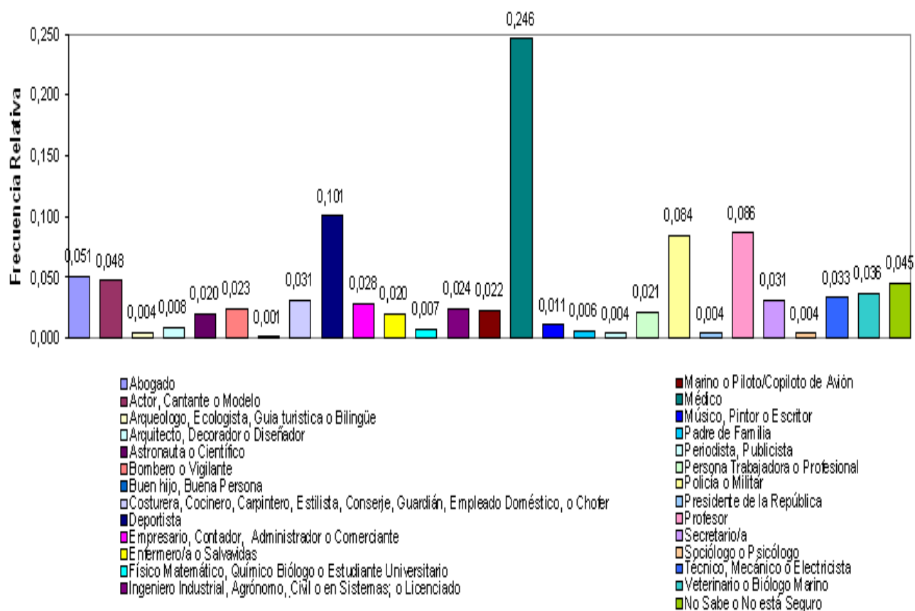
Histograma de Frecuencias
