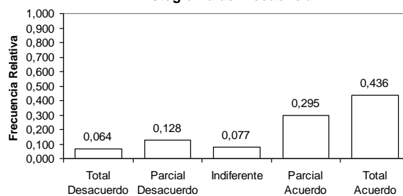
Histograma de Frecuencia
