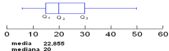
Diagrama de Caja sin valores aberrantes
