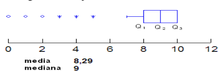
Diagrama de Caja con valores aberrantes
