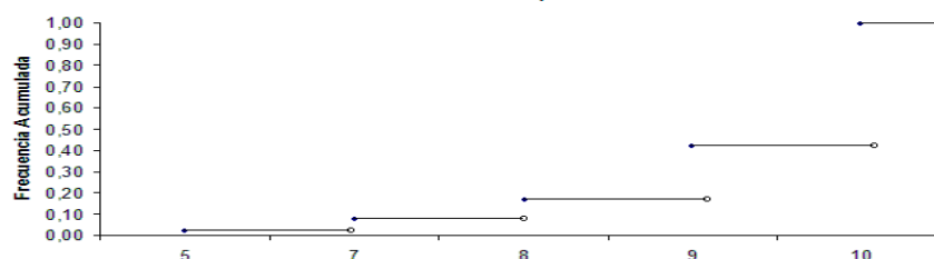
Distribución Empírica
