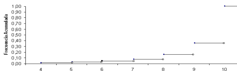
Distribución Empírica
