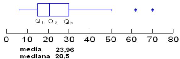
Diagrama de Caja con valores aberrantes
