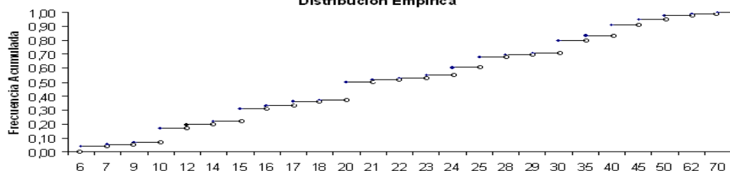
Distribución Empírica
