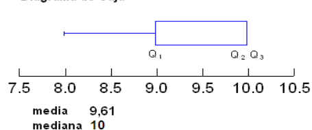
Diagrama de Caja sin valores aberrantes
