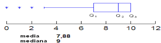
Diagrama de Caja con valores aberrantes
