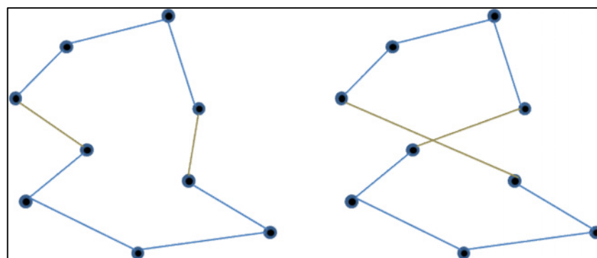
Figura 2.4. Ejemplo de intercambio 2 opt
