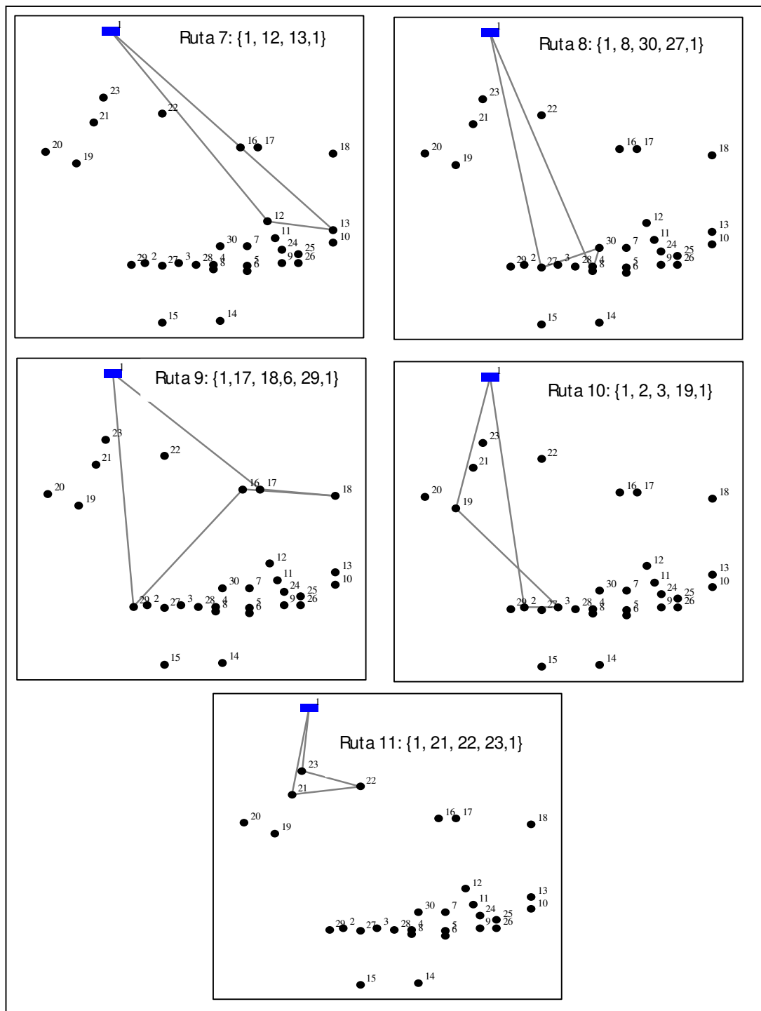
Figura 3.4. Rutas individuales del ruteo vehicular parte 2
