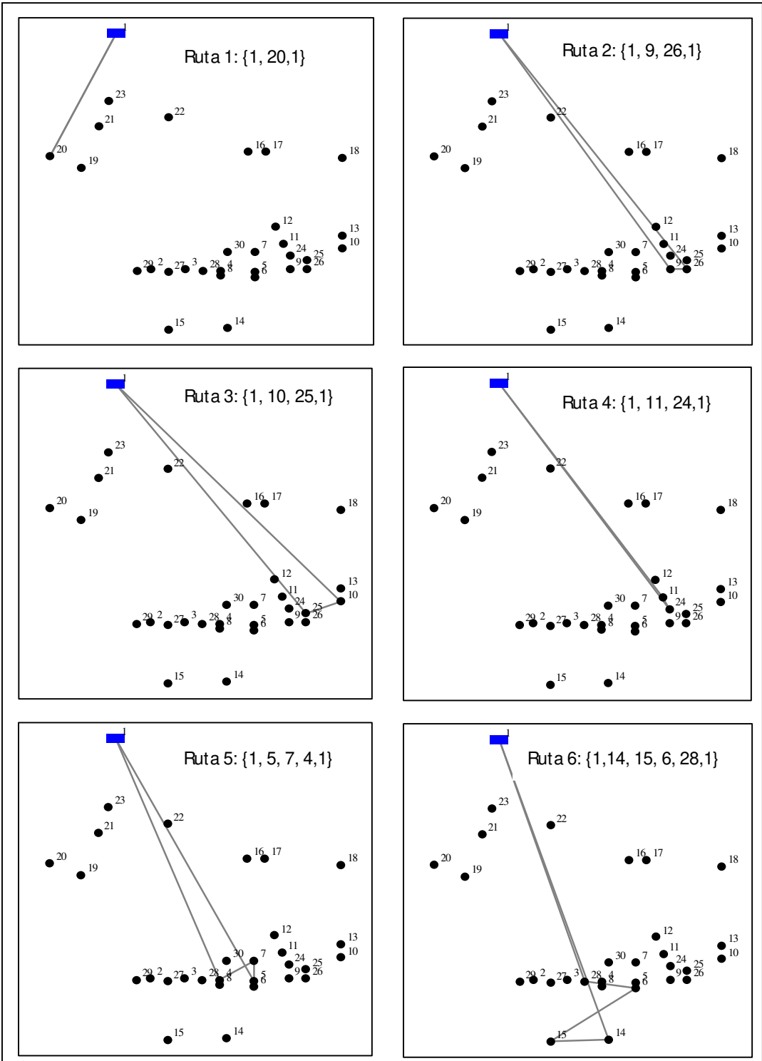
Figura 3.3. Rutas individuales del ruteo vehicular parte 1
