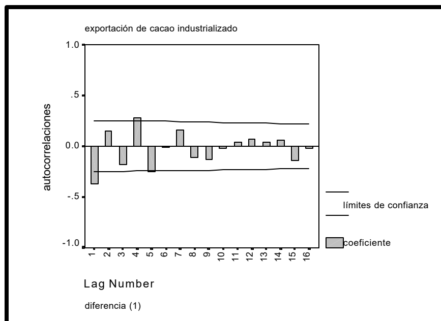
FIGURA 3.58 AUTOCORRELACIONES
