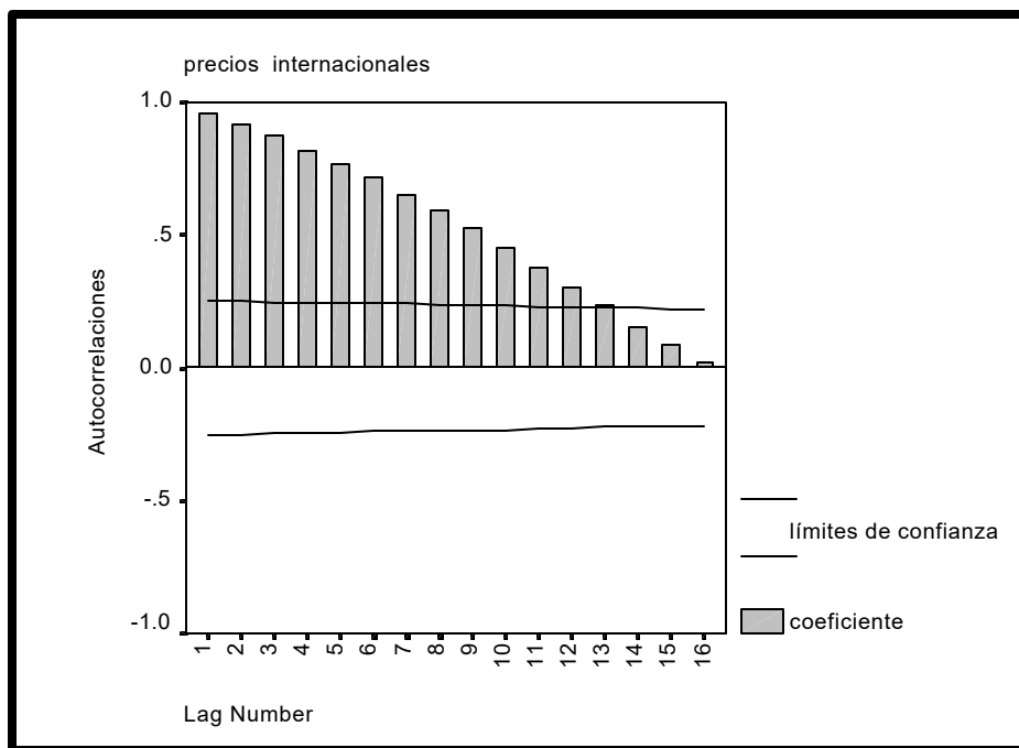
FIGURA 3.63 AUTOCORRELACIONES
