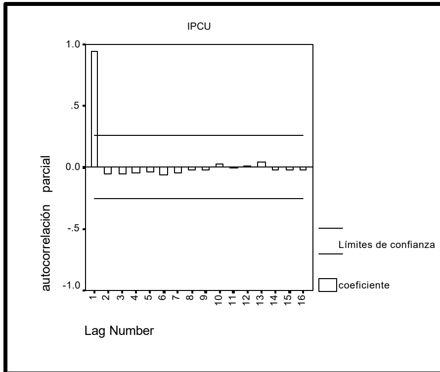
FIGURA 3.73 AUTOCORRELACIONES PARCIALES
