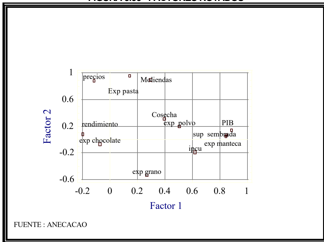
FIGURA 3.35 FACTORES ROTADOS
