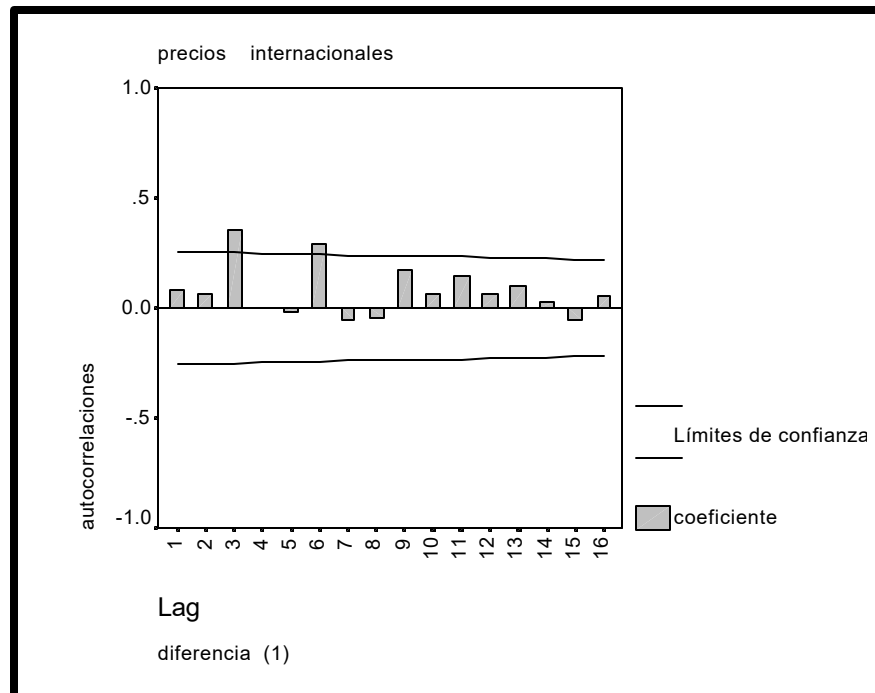
FIGURA 3.66 AUTOCORRELACIONES
