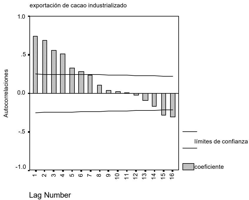
FIGURA 3.55 AUTOCORRELACIONES
