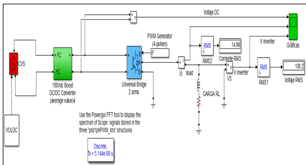
Figura 5.13 Inversor AC - Elaboración Propia
