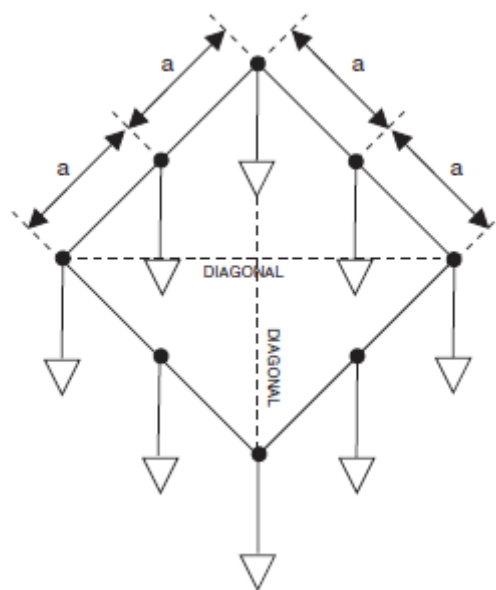
Figura 3. 4 Método de electrodos múltiples
