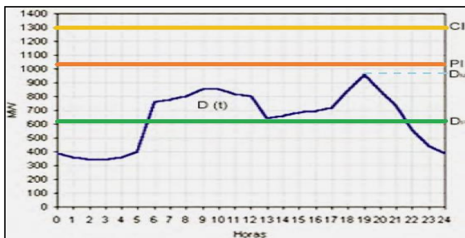
Figura 1.9 Curva de Carga Diaria Típica [1]
