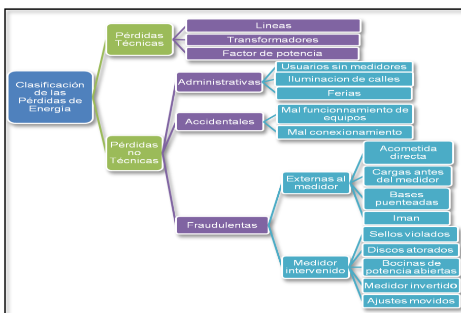
Figura 1.11 Clasificación de las Pérdidas de Energía
