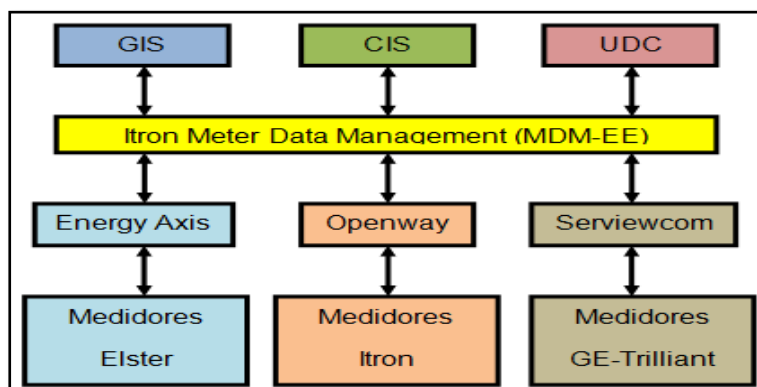
Figura 1.13 Diagrama de bloques de la arquitectura AMI implementada en la CNEL-Guayaquil
