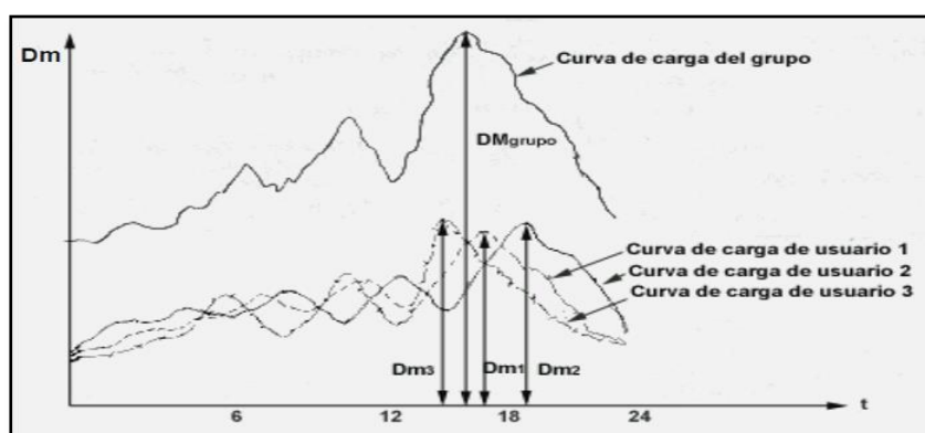
Figura 1.10 Curvas de carga de diferentes usuarios y la curva de carga equivalente del grupo [1]
