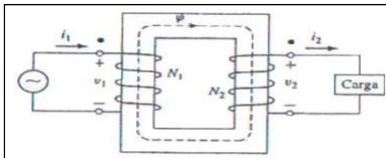
Figura 1.2 Transformador de dos Devanados [6]
