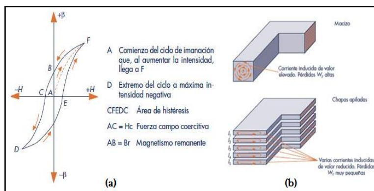
Figura 1.12 (a) Ciclo de Histéresis y (b) Corrientes Parásitas Presentes en un Transformador [14]
