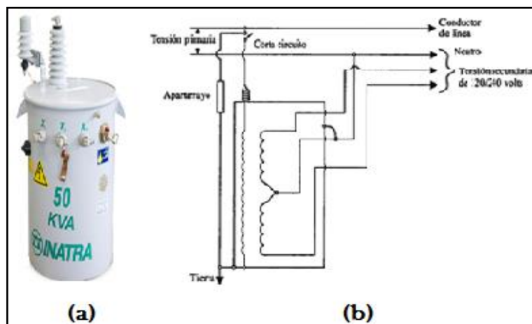
Figura 1.5 (a) Transformador monofásico convencional tipo poste y (b) Esquema Funcional del Transformador [8]
