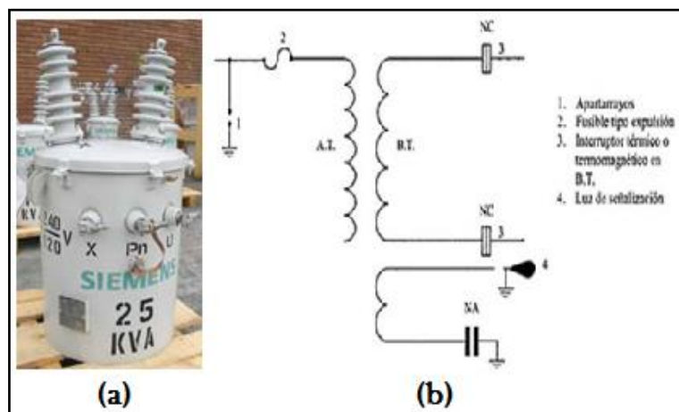
Figura 1.6 (a) Transformador Monofásico Autoprotegido Tipo Poste y (b) Esquema Funcional del Transformador [8]
