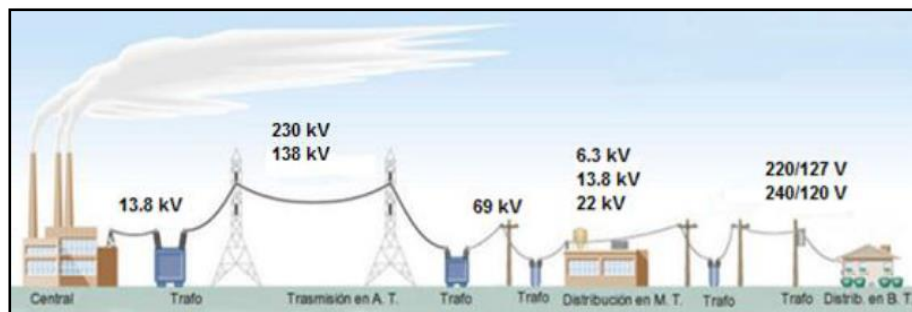
Figura 1.1 Esquema Básico de un Sistema Eléctrico de Potencia [2]
