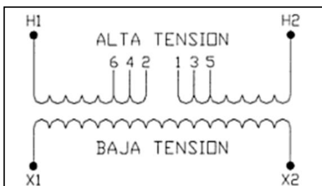
Figura 1.4 Esquema Funcional de un Transformador de Distribución Monofásico [8]
