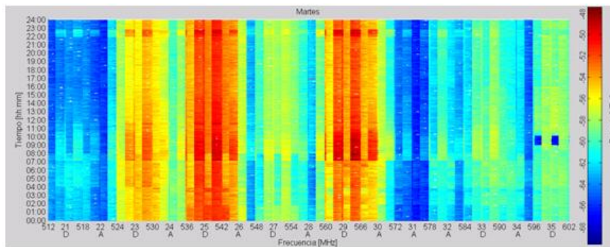
Figura 4.6 Utilización del espectro martes 00:00 a 24:00 Frecuencias 512 – 602MHz
