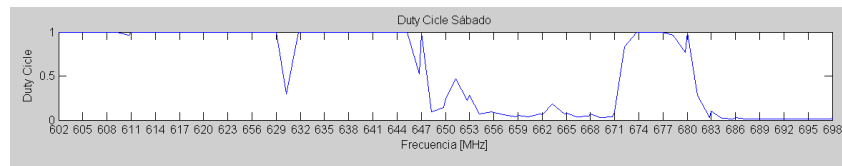
Figura 4.25 Duty cycle sábado 00:00 a 24:00 Frecuencias 602– 698MHz
