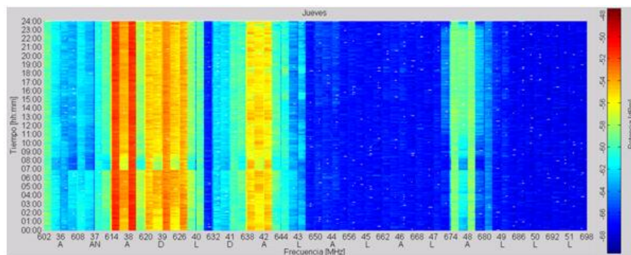
Figura 4.16 Utilización del espectro jueves 00:00 a 24:00 Frecuencias 602 – 698MHz
