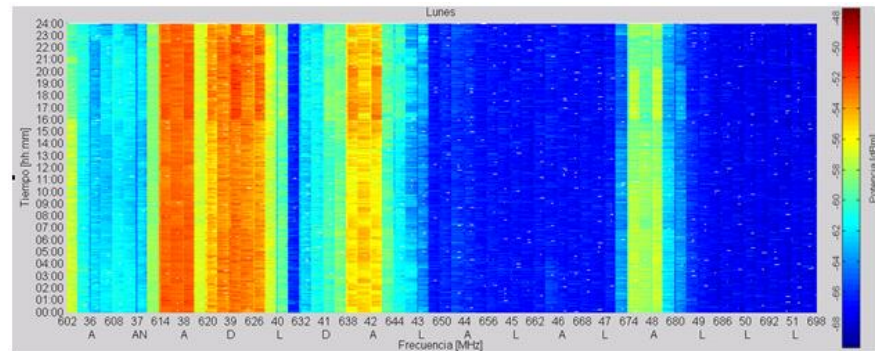
Figura 4.4 Utilización del espectro lunes 00:00 a 24:00 Frecuencias 602 – 698MHz
