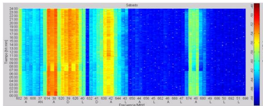
Figura 4.24 Utilización del espectro sábado 00:00 a 24:00 Frecuencias 602 – 698MHz
