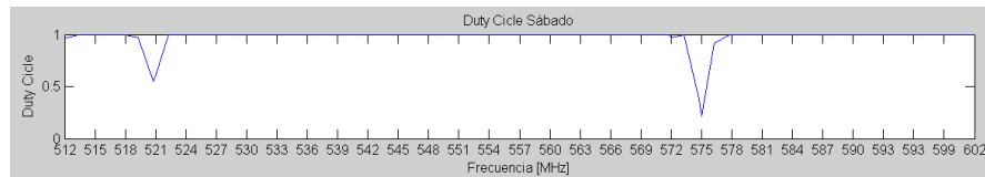
Figura 4.23 Duty cycle sábado 00:00 a 24:00 Frecuencias 512 – 602MHz
