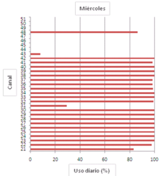
Figura 4.32 Porcentaje de uso por canal Miércoles
