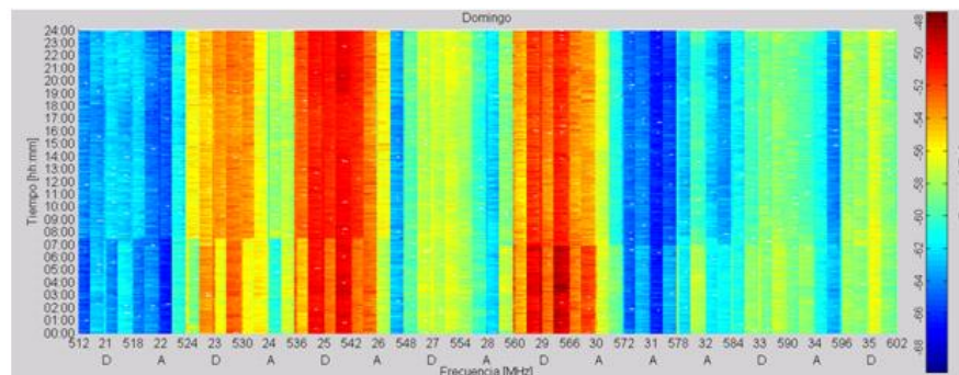
Figura 4.26 Utilización del espectro domingo 00:00 a 24:00 Frecuencias 512 – 602MHz
