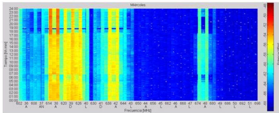
Figura 4.12 Utilización del espectro miércoles 00:00 a 24:00 Frecuencias 602 – 698MHz
