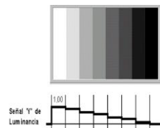
Figura 2.5 Señal de Luminancia, escala de grises [10]
