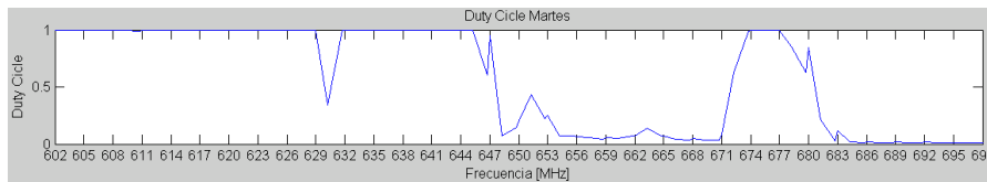
Figura 4.9 Duty cycle martes 00:00 a 24:00 Frecuencias 602– 698MHz
