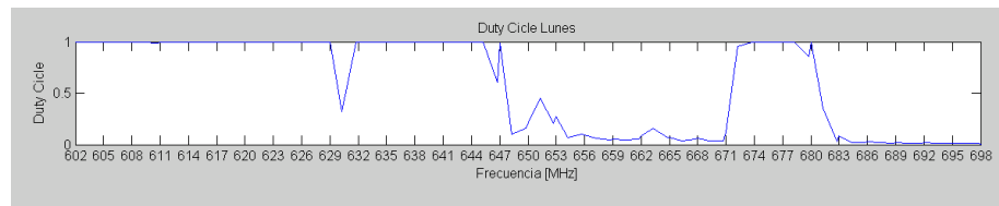
Figura 4.5 Duty cycle lunes 00:00 a 24:00 Frecuencias 602– 698MHz
