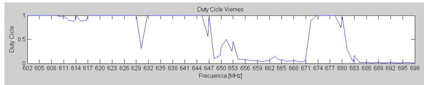
Figura 4.21 Duty cycle viernes 00:00 a 24:00 Frecuencias 602– 698MHz
