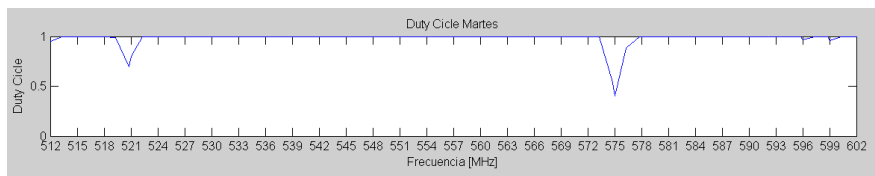
Figura 4.7 Duty cycle martes 00:00 a 24:00 Frecuencias 512 – 602MHz
