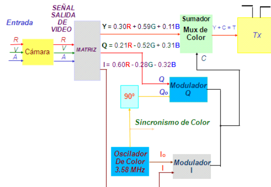
Figura 2.6 Modulación de Señal Y [10]
