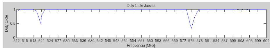
Figura 4.15 Duty cycle jueves 00:00 a 24:00 Frecuencias 512 – 602MHz
