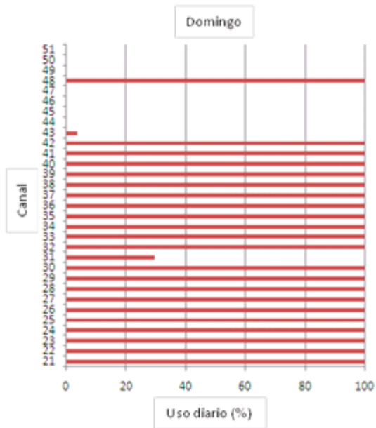
Figura 4.36 Porcentaje de uso por canal Domingo
