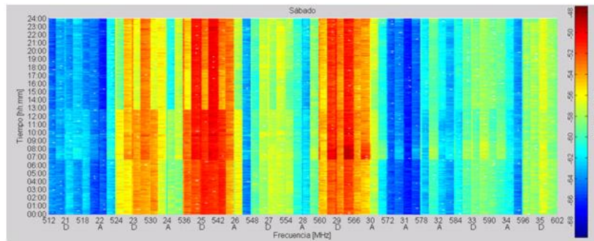
Figura 4.22 Utilización del espectro sábado 00:00 a 24:00 Frecuencias 512 – 602MHz
