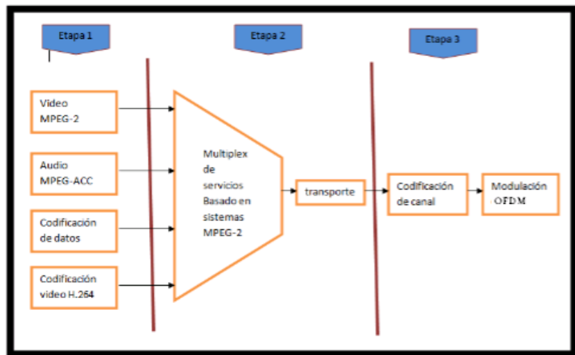
Figura 2.10 Modelamiento SBTVD [12]
