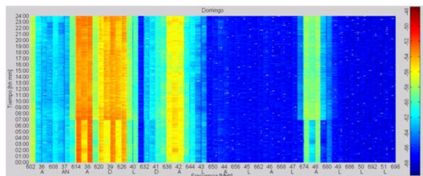
Figura 4.28 Utilización del espectro domingo 00:00 a 24:00 Frecuencias 602 – 698MHz
