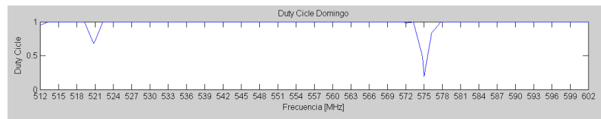
Figura 4.27 Duty cycle domingo 00:00 a 24:00 Frecuencias 512 – 602MHz
