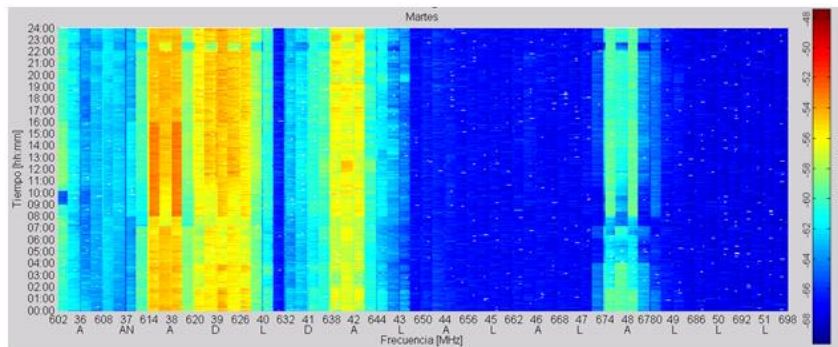
Figura 4.8 Utilización del espectro martes 00:00 a 24:00 Frecuencias 602 – 698MHz
