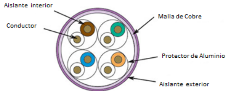
Figura 1.1: Cable tipo S/FTP categoría 6A.
