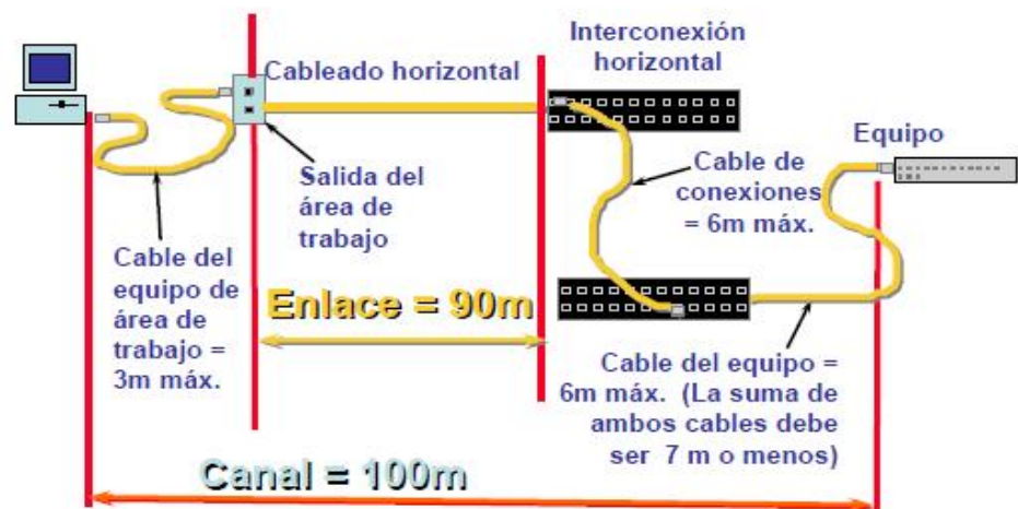
Figura 1.2: Instalación del cableado horizontal.
