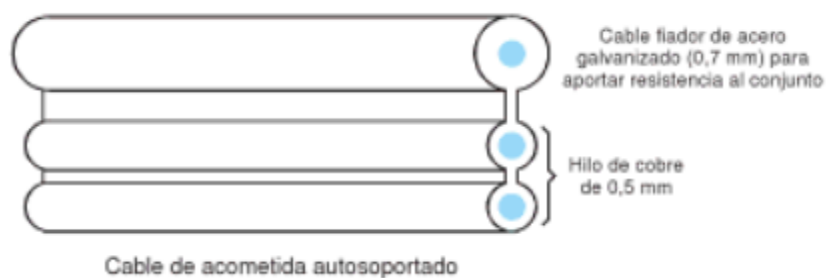
Fig.13.14 CABLE DE ACOMETIDA AUTOSOPORTADO[15]
