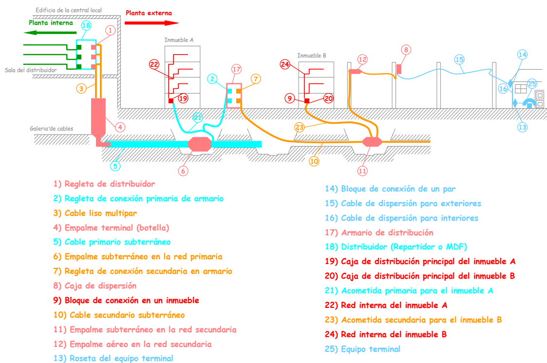
FIG.5.6 COMPONENTES DE LA PLANTA EXTERNA[14]
