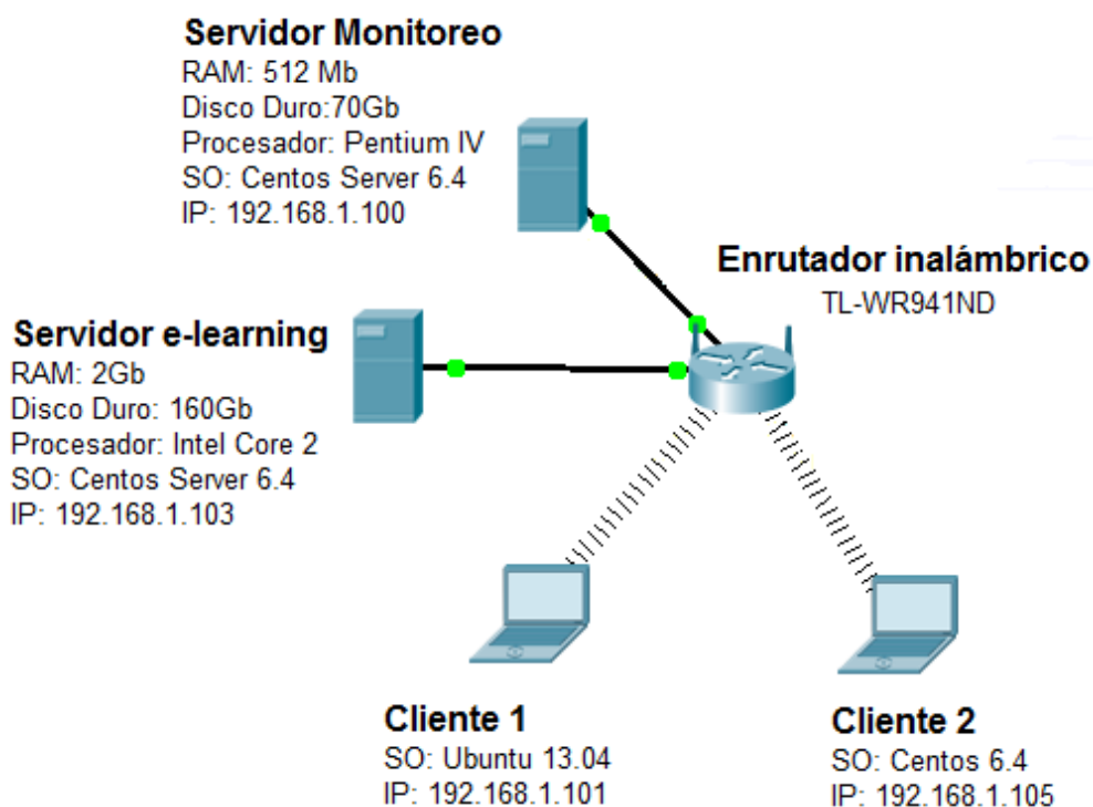
Figura 3-1 Topología de la Red
