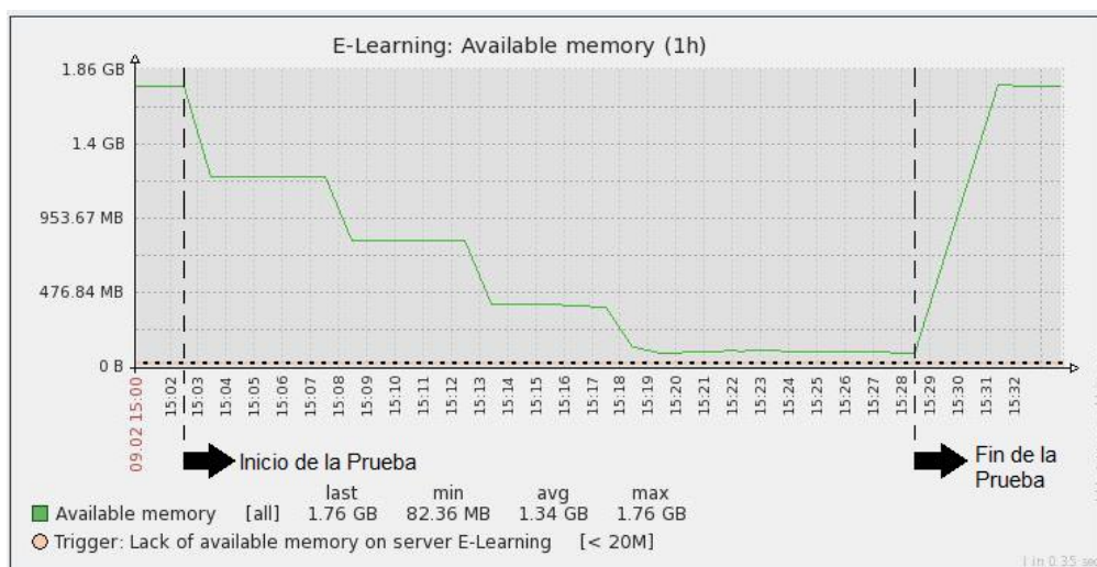
Figura 4-1 Consumo de Memoria RAM Moodle
