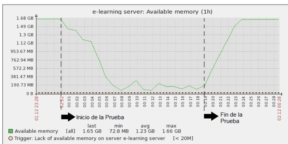
Figura 4-2 Consumo de Memoria RAM Claroline
