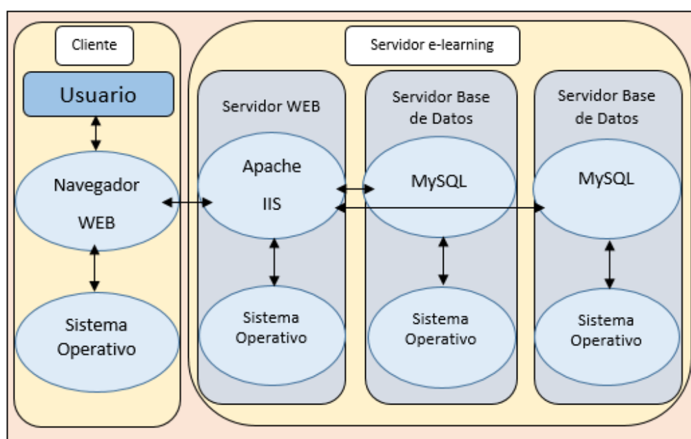
Figura 2–3: Diagrama de Despliegue de Claroline. [1]
