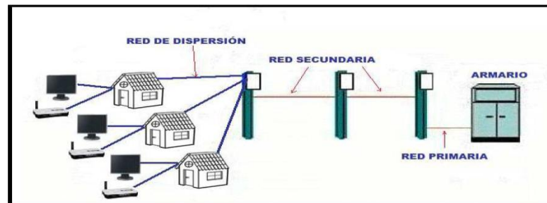
Figura 3.3 Elementos Principales Planta Externa
