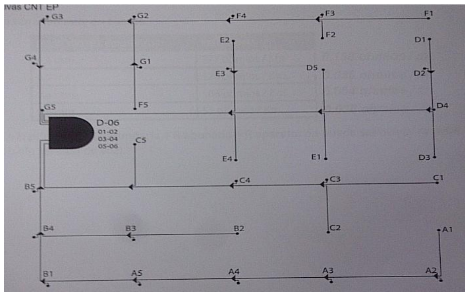
Figura 3.26 Diagrama Red Secundaria
