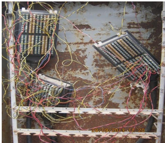
Figura 3.23 Regletas en Armario 02
