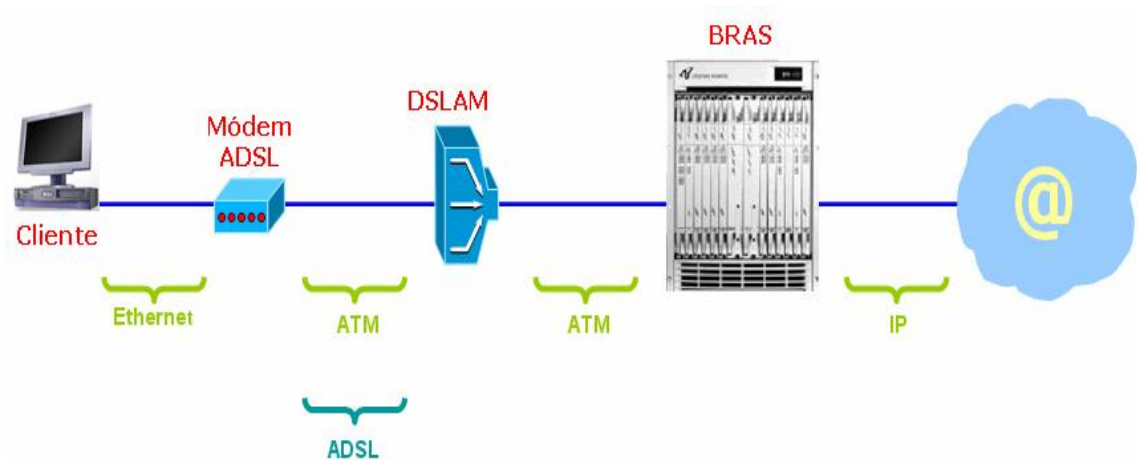
Figura 2.1 Modelo de Acceso a Internet
