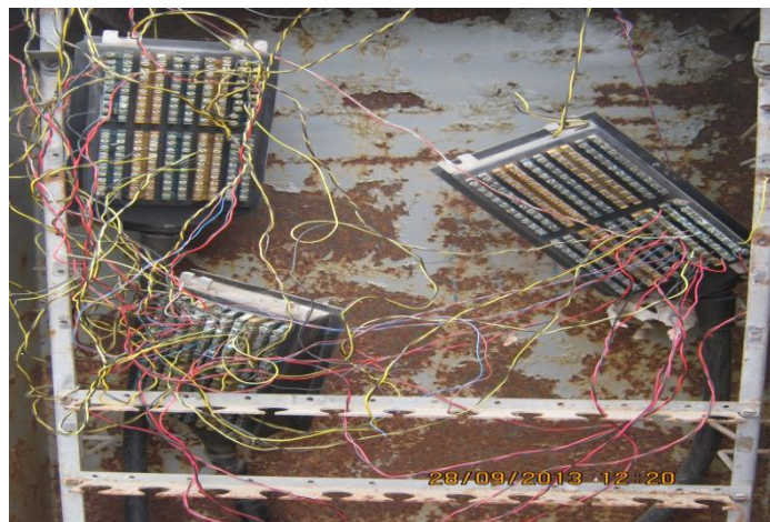
Figura 4.2 Regletas Primaria y Secundaria
