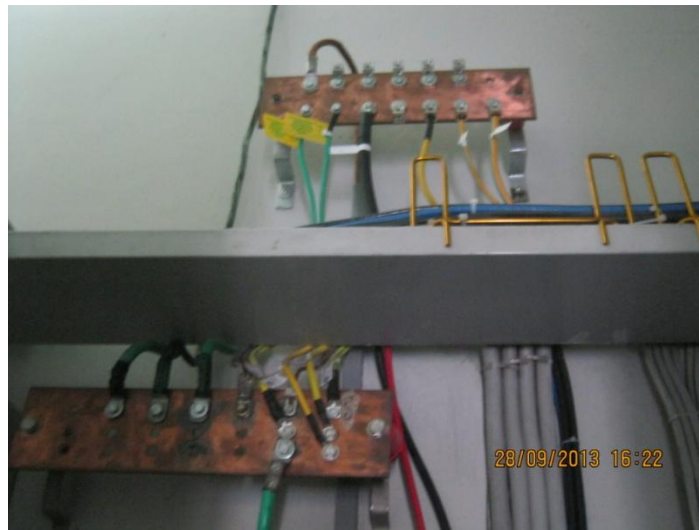
Figura 3.19 Conexión a Tierra (Cuarto de Baterías)
