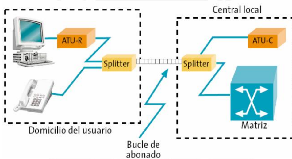
Figura 2.5 Diseño de Red ADSL
