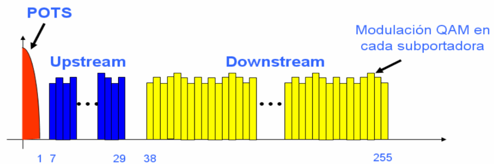
Figura 2.3 Modulación DMT.
