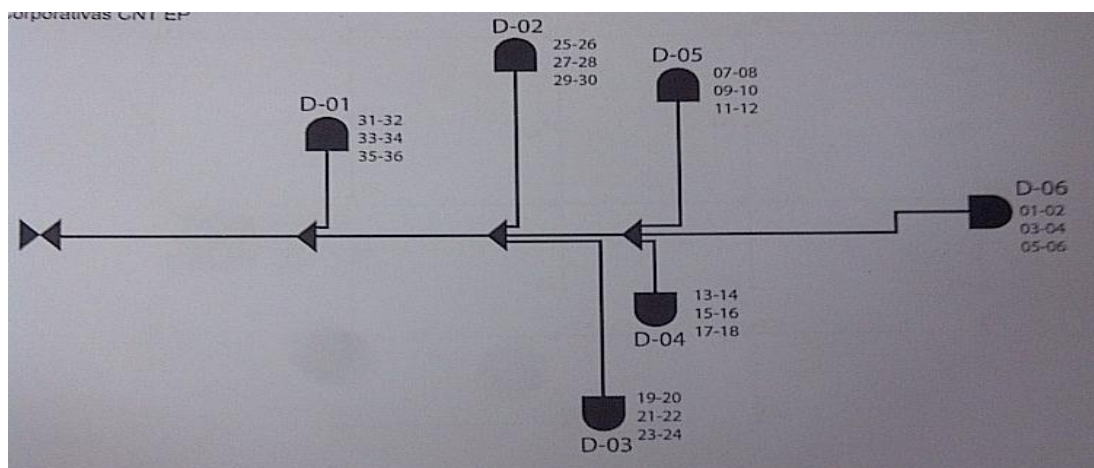
Figura 3.20 Diagrama Red Primaria
