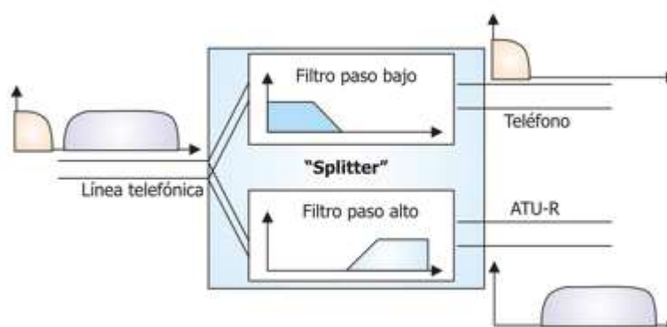
Figura 2.8: Funcionamiento del Splitter [16]
