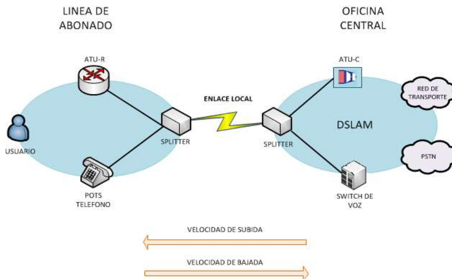
Figura 2.7: Arquitectura de una red ADSL2 [18]
