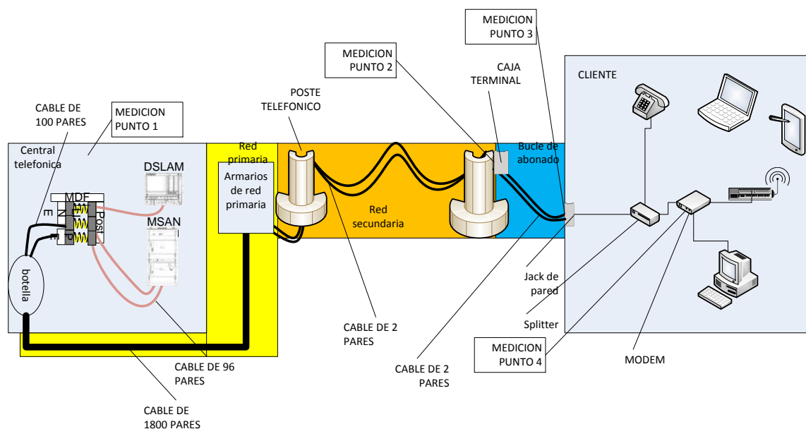
Figura 5.19: Diagrama de mediciones
