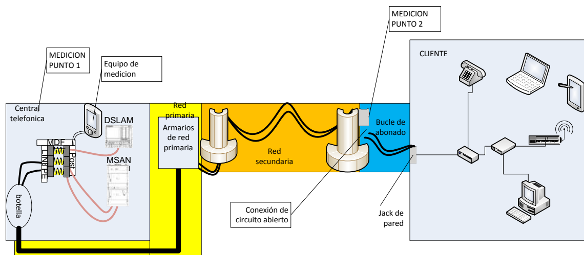
Figura 5.23: Medición de balance longitudinal en un par de cobre [18]
