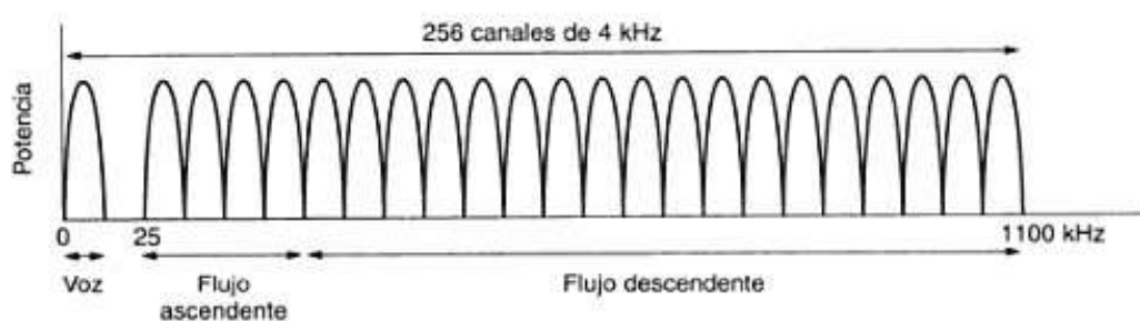
Figura 2.5: ADSL con Modulación discreta.
