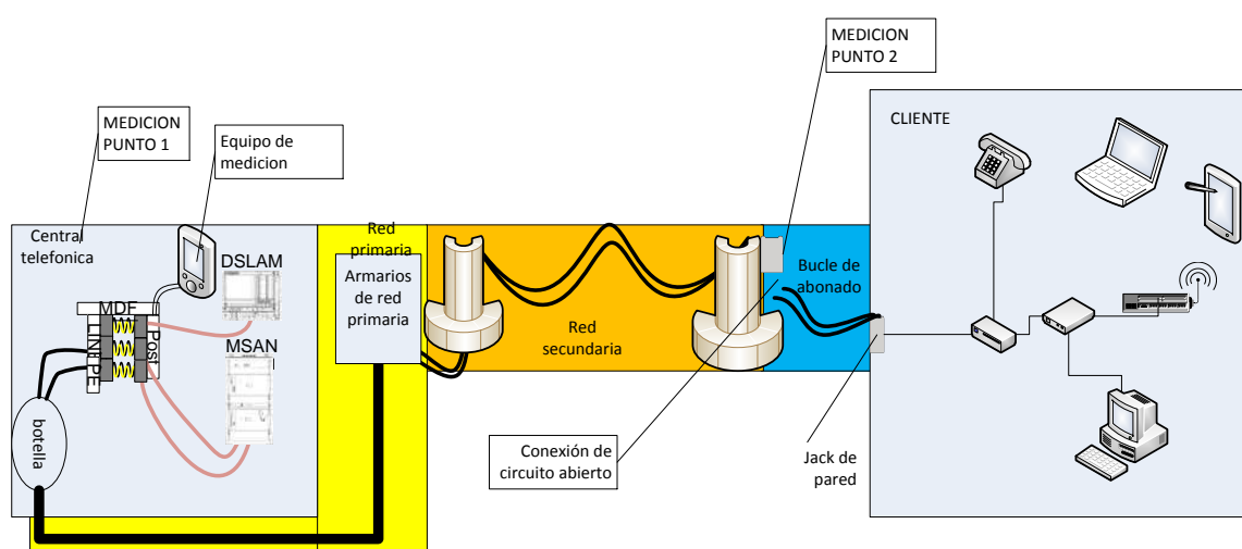
Figura 5.21: Medición de aislamiento en un par de cobre [18]
