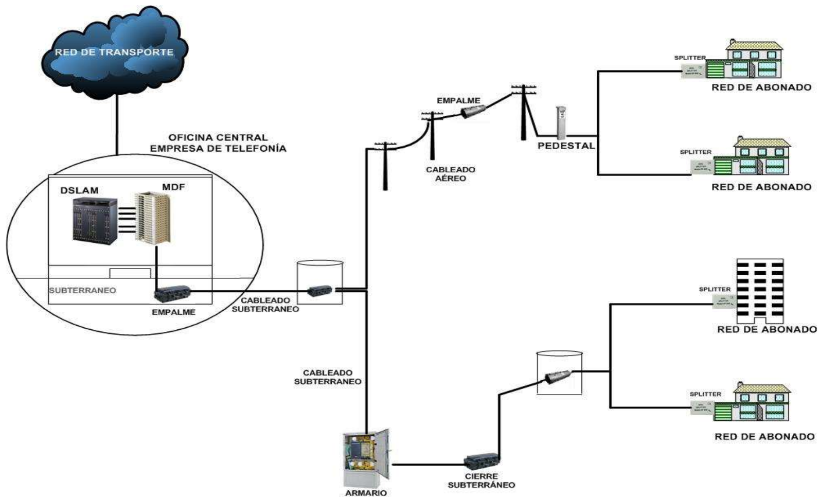
Figura 6.25: Diseño Lógico de la red
