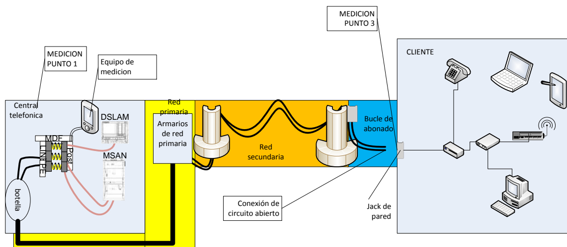
Figura 5.22: Medición de longitud de línea en un par de cobre [18]
