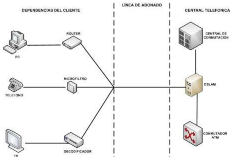
Figura 2.1: Elementos de una red xDSL [17]
