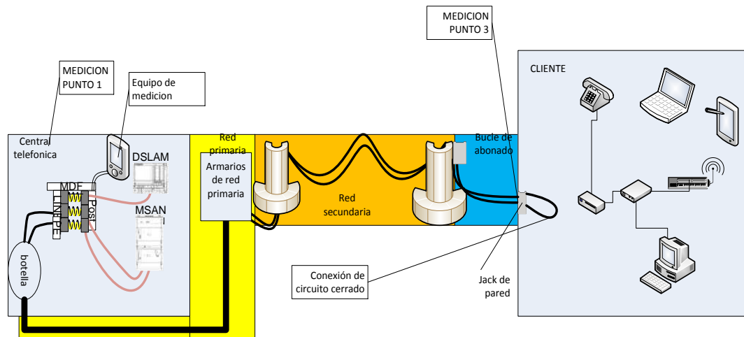
Figura 5.20: Medición de resistencia en un par de cobre [18]
