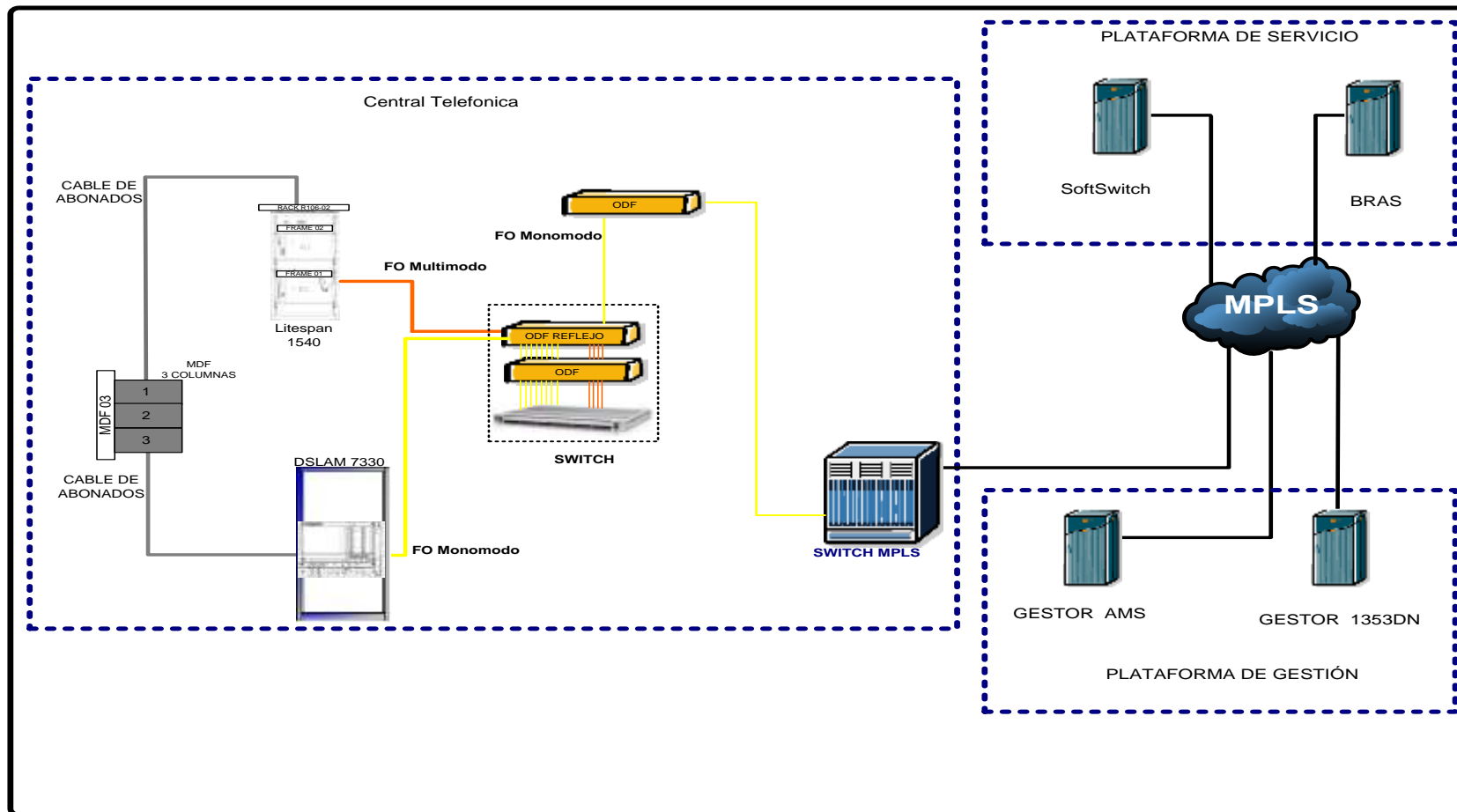
Figura 4.10: Topología de conexión de red [18]
