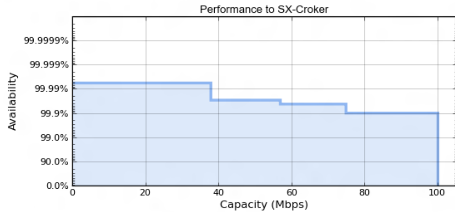
Figura 6. 14: Disponibilidad y ancho de banda simulado.
