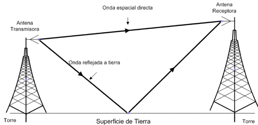
Figura 2. 9: Propagación de ondas espaciales [7].
