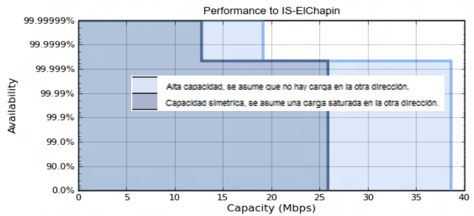
Figura 6. 16: Disponibilidad y ancho de banda simulado.
