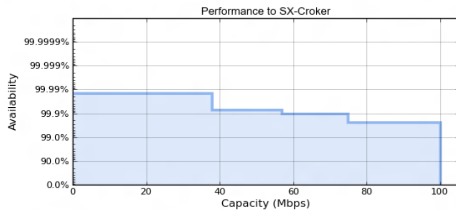
Figura 6. 12: Disponibilidad y ancho de banda simulado.
