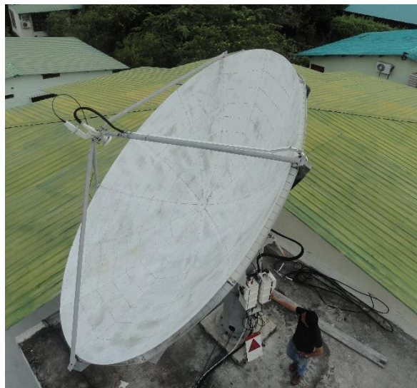
Figura 3. 3: Antena de foco central DPNG-Santa Cruz.
