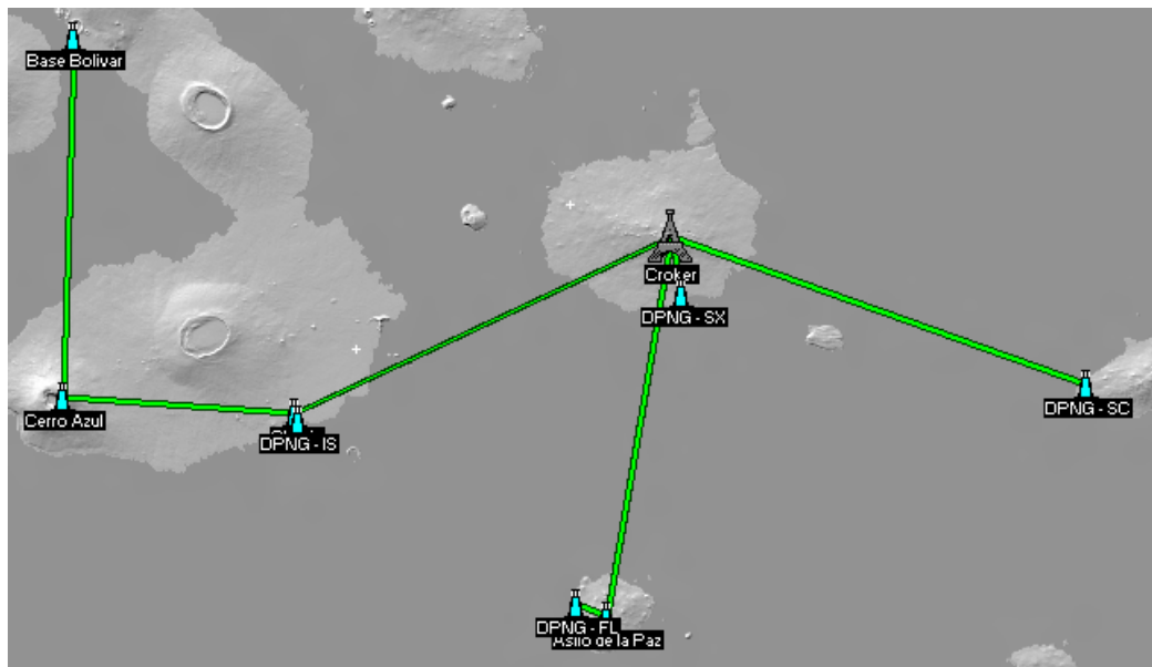
Figura 6. 1: Estructura de red.
