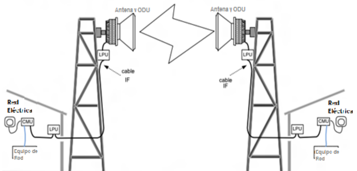
Figura 4. 2: Componentes de red, solución PTP Cambium Networks. [21].
