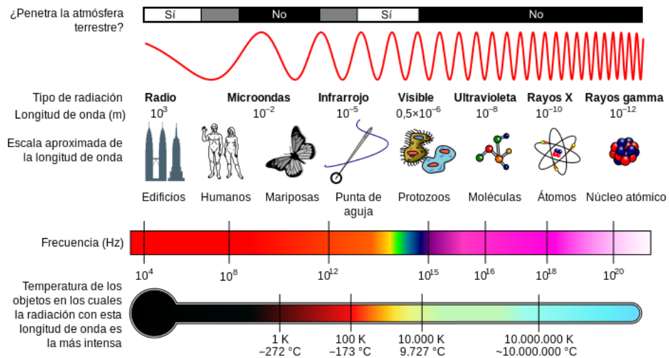
Figura 2. 8: Diagrama del espectro electromagnético, mostrando el tipo, longitud de onda (con ejemplos), frecuencia y la temperatura de emisión de cuerpo negro [6].
