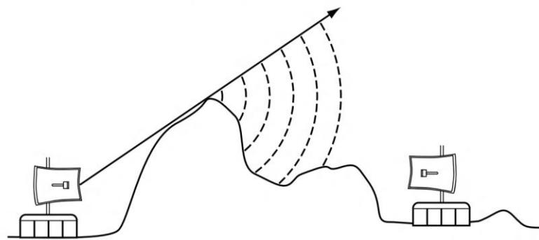
Figura 2. 6: Difracción en la cima de una montaña. [3].
