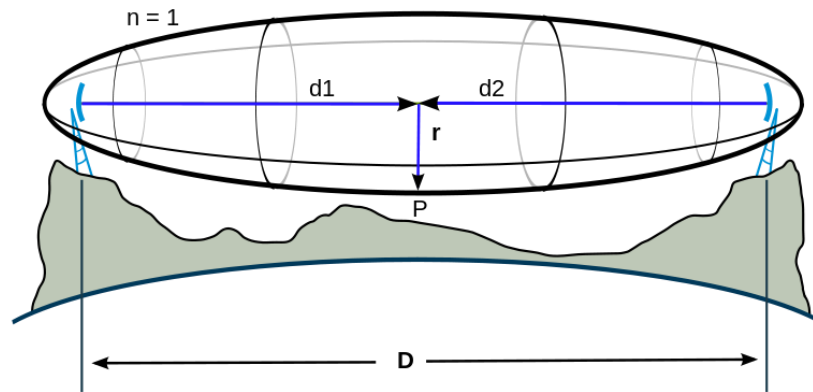
Figura 2. 10: Zonas de Fresnel [10].
