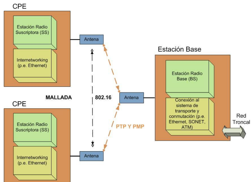
Figura 4. 1: Conexión entre SS y BS [19].
