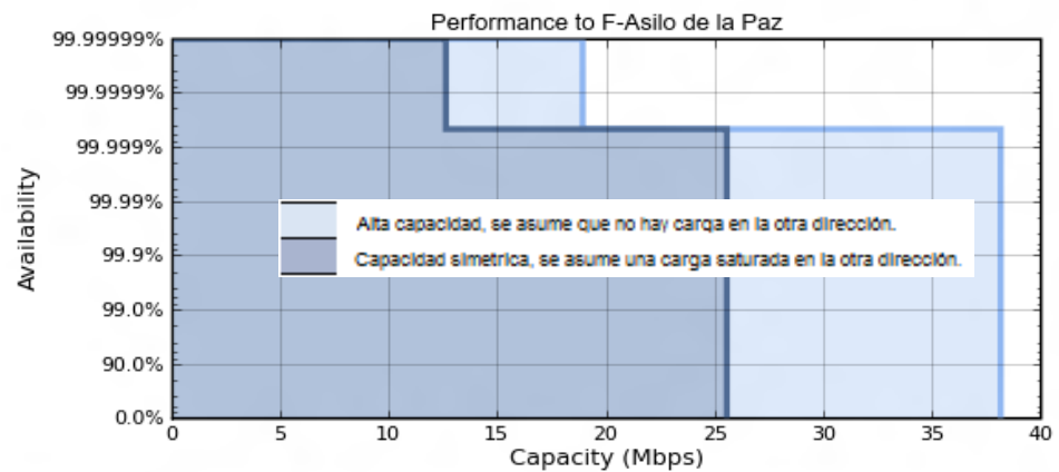
Figura 6. 10: Disponibilidad y ancho de banda simulado.
