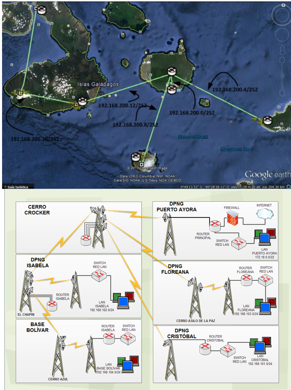
Figura 6. 21: Diagrama de red WAN para la DPNG.
