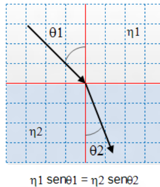
Figura 2. 5: Refracción de una onda. [4].
