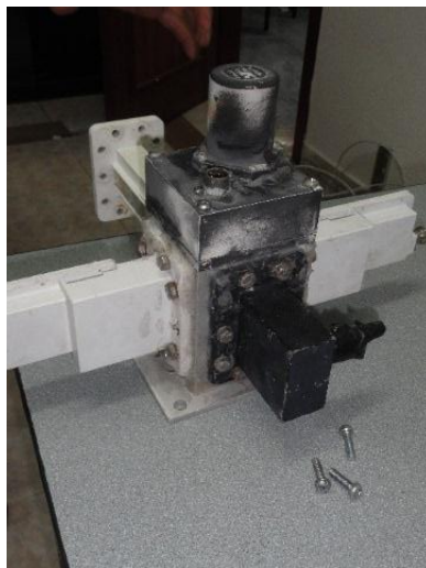
Figura 3. 4: Sistema de conmutación automático entre LNA y transceptor.
