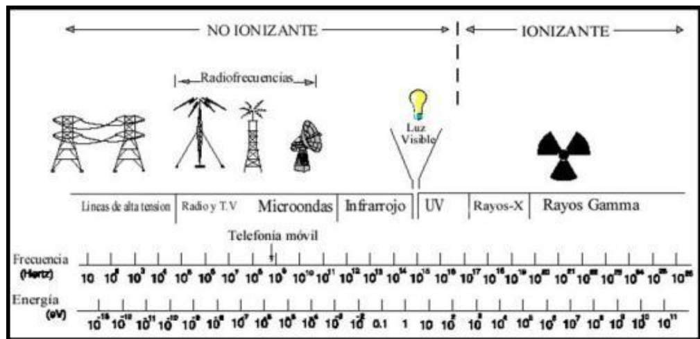
Figura 6. 2: Espectro Electromagnético. [24]
