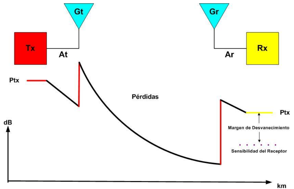
Figura 6. 4: Presupuesto de Enlace.
