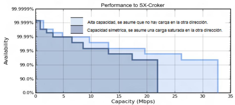
Figura 6. 8: Disponibilidad y ancho de banda simulado.
