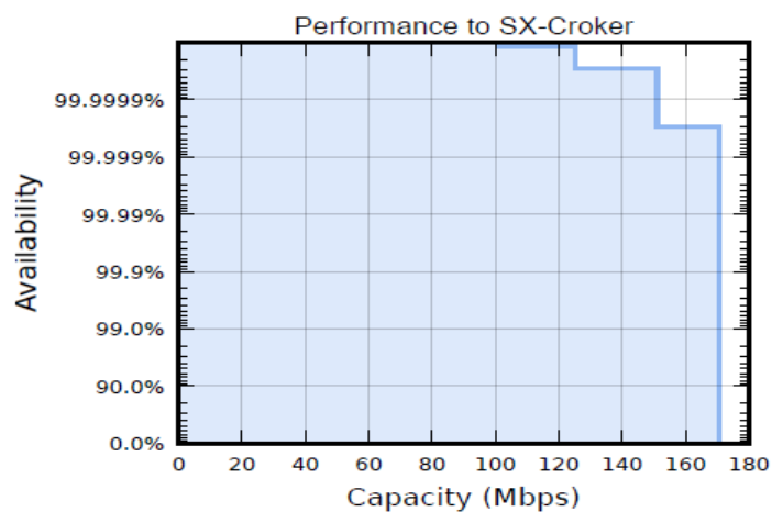
Figura 6. 6: Disponibilidad y ancho de banda simulado.
